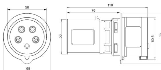
Dimensiones en mm / Dimensions in mm
