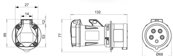
Dimensiones en mm / Dimensions in mm
