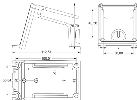
Dimensiones en mm / Dimensions in mm
