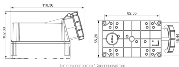
Dimensiones en mm / Dimensions in mm
