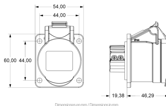
Dimensiones en mm / Dimensions in mm
