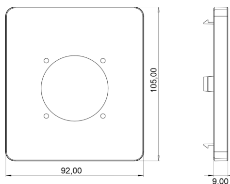
Dimensiones en mm / Dimensions in mm
