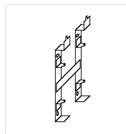
Soporte de pared en forma de H.
