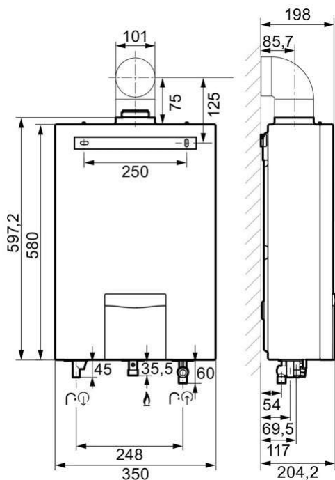
Dimensiones (mm)
