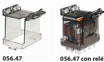
Adaptador con aletas en carril 35 mm (EN 60715) en la parte superior para relé tipo 56.34
