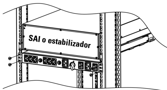
Montaje en rack de 19"
