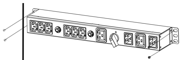
Montaje mural.
