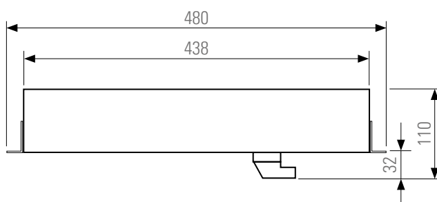
Fig. 9. Dimensiones BM-R 3 kVA.
