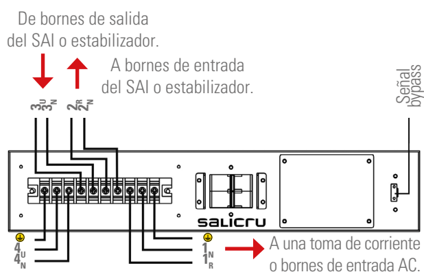
Fig. 8. Ejemplo conexionado bypass manual de 6 y 10 kVA.
