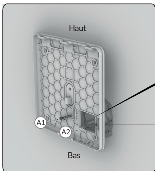
Boîte d'encastrement
