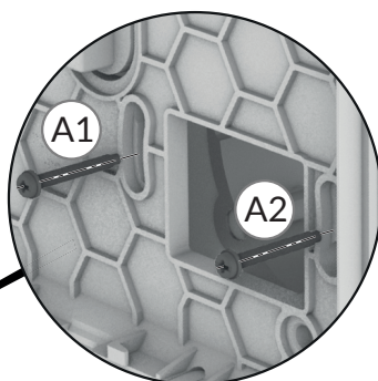
Boîte d'encastrement
