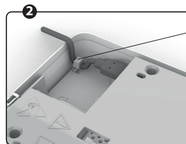
Cable gland
