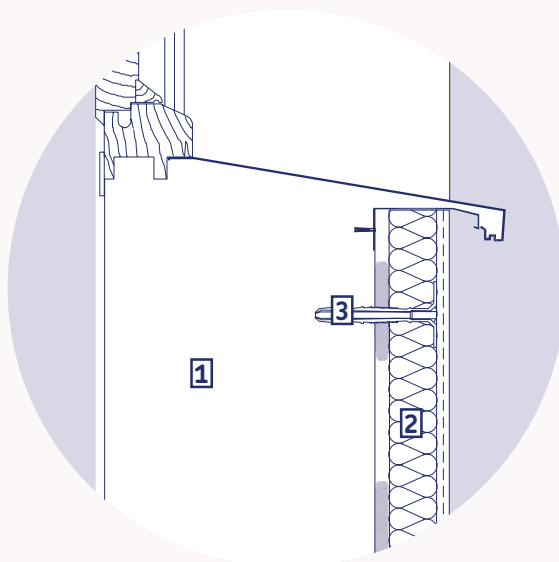
1 Soporte 2 URSA XPS 3 Fijación
