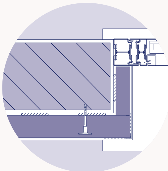
Detalle ventana
