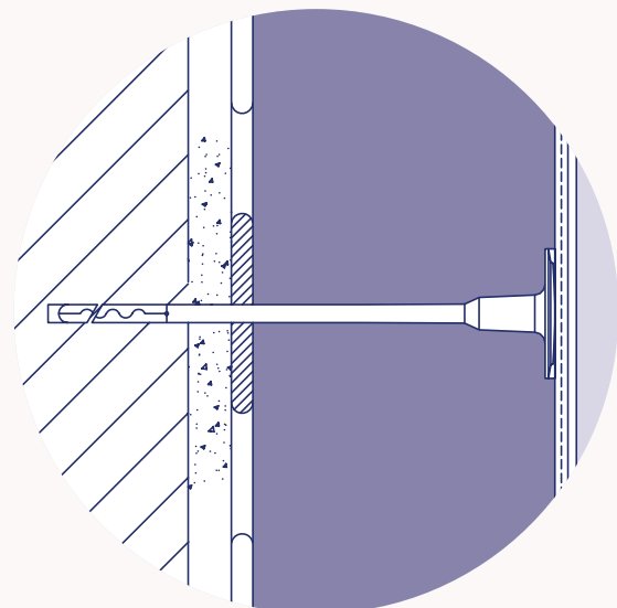
Detalle de anclaje con fijación plástica.
