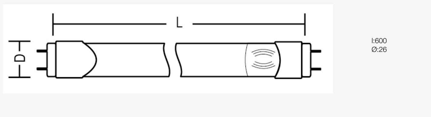
Esquema de Producto. Product line drawing
