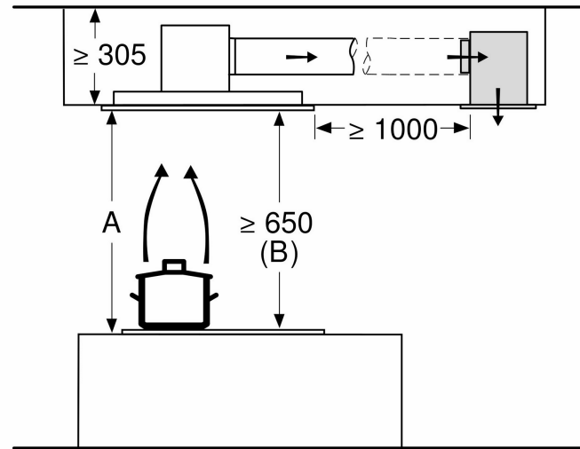
Dimensiones en mm Circulación de aire
