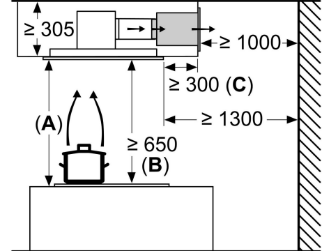
Dimensiones en mm Circulación de aire
