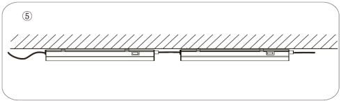
Diagrama de instalación del tubo acoplable, cantidad máx. acoplable con 30 unidades
