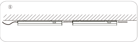
Diagrama de instalação do tubo de acoplamento, quantidade máxima de acoplamento com 30 unidades
