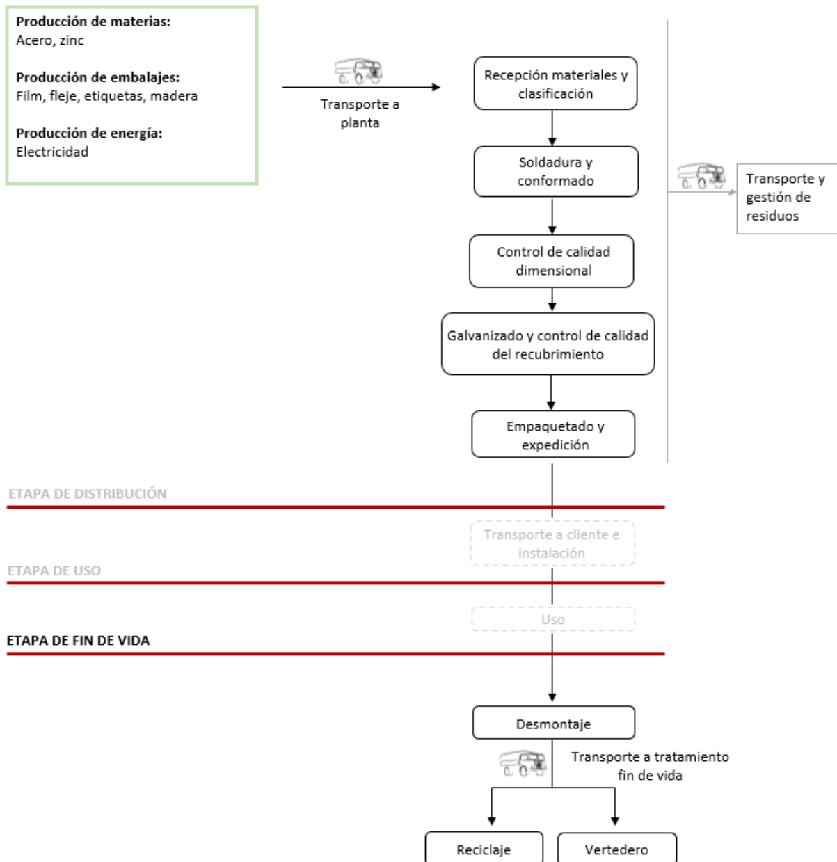
Imagen 1 Diagrama de proceso de producción.
