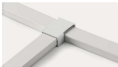
Ángulo "T" Troquele las paredes B y C
