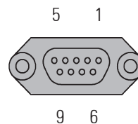
Fig. 3. Connecteur interface RS-232, (X31).
