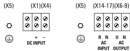
Modelo IS-B (con línea de bypass estático). IS-B model (with static bypass line). Modèle IS-B (avec ligne de bypass statique).
