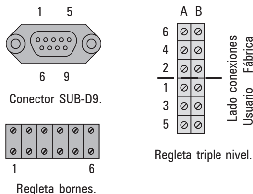
Fig. 2. Interface a relés, (X32).
