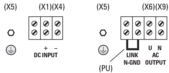
Modelo básico (sin línea de bypass estático). Basic model (no static bypass line). Modèle basique (sans ligne de bypass statique).
