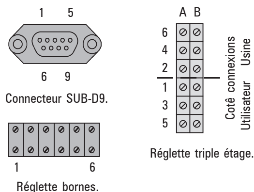
Fig. 2. Interface à relais, (X32).
