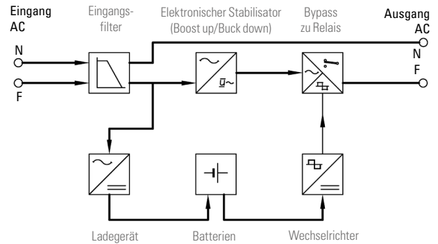
Fig. 2. Strukturelles Blockschema.
