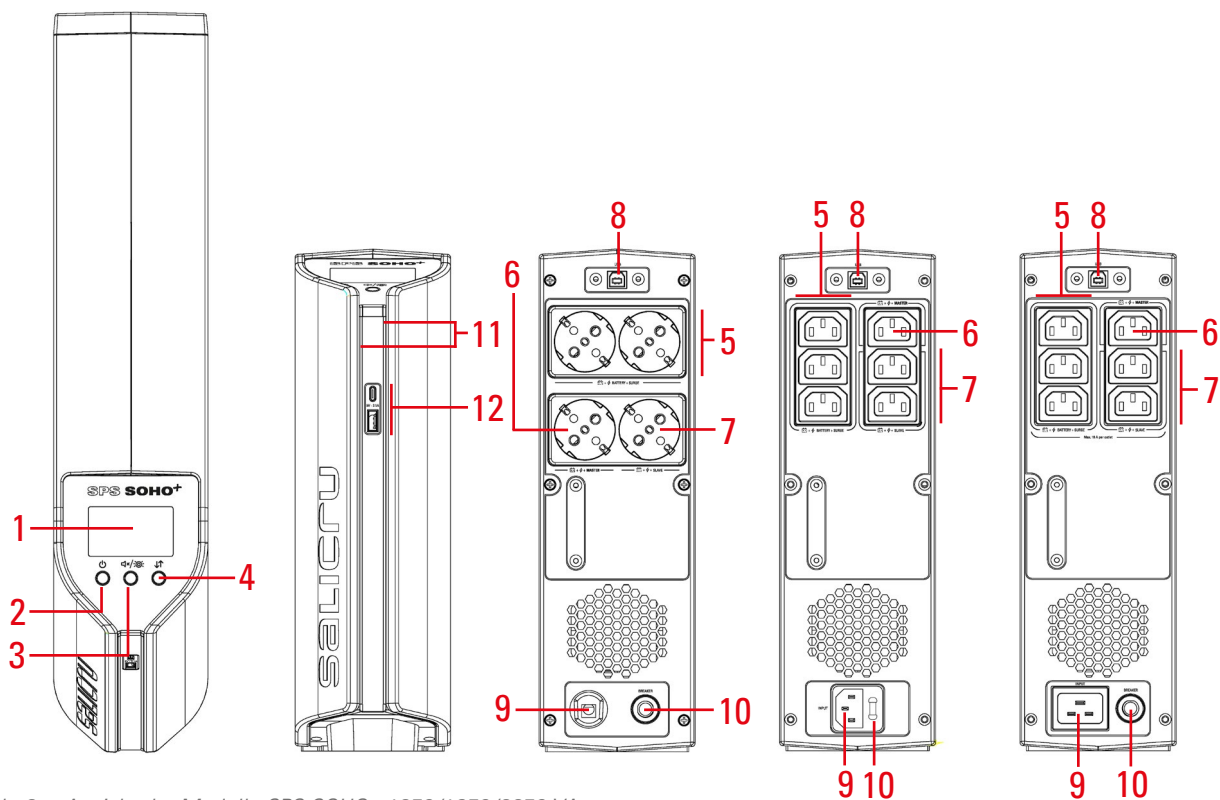
Abb. 2. Ansicht der Modelle SPS SOHO+ 1250/1650/2250 VA.
