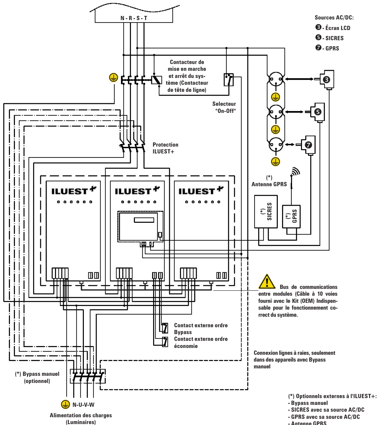
Fig. 20. Schéma connexion exécution (OEM) triphasé.
