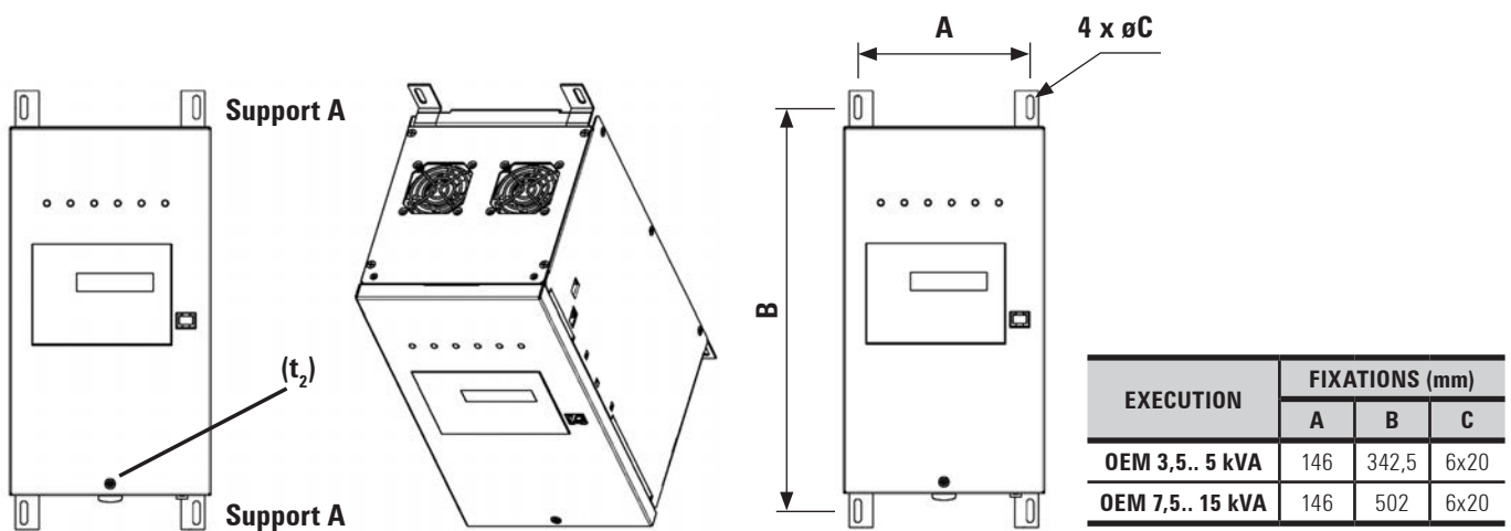
Fig. 14. Plan fixation module exécution (OEM).
