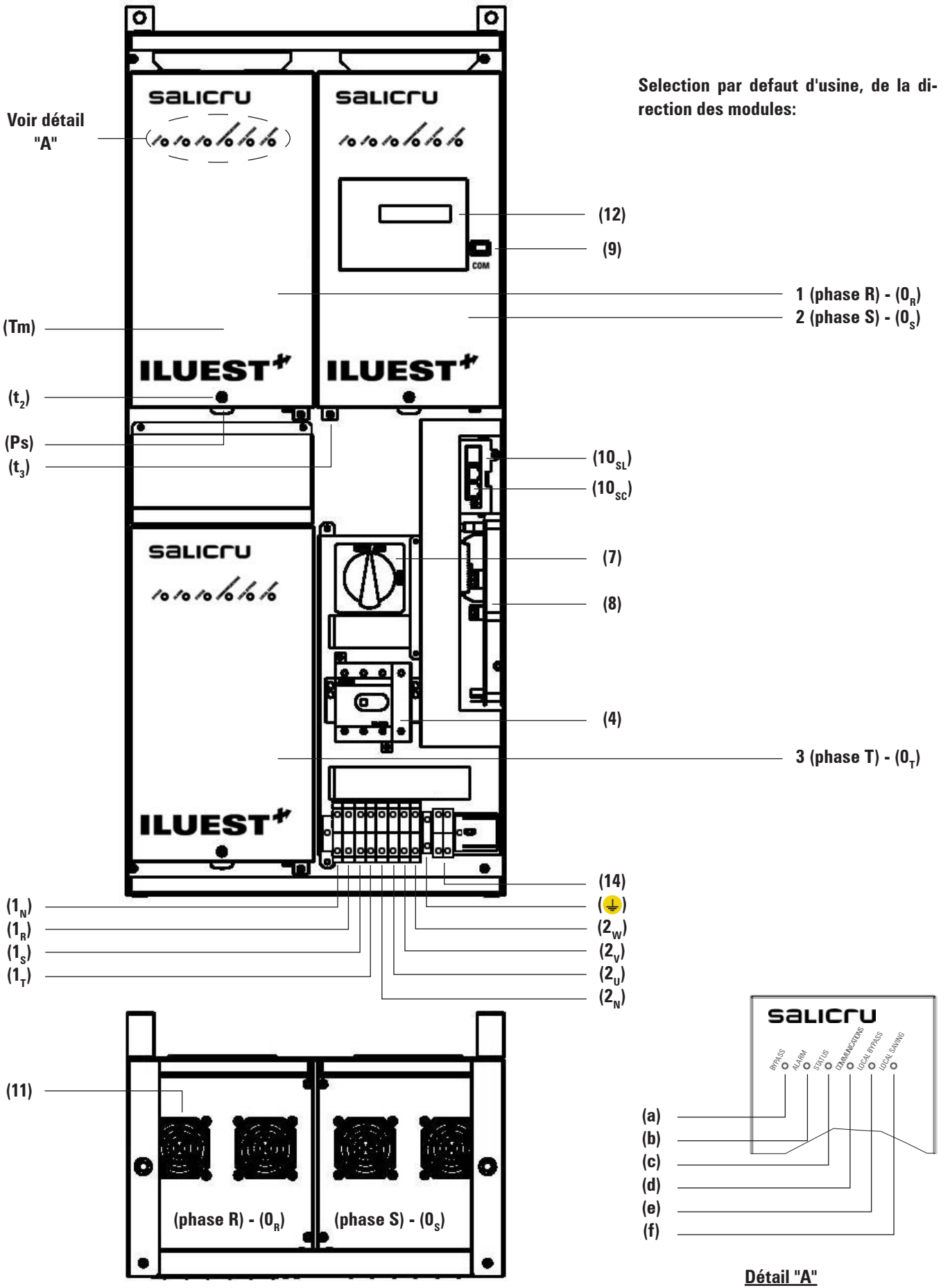
Fig. 5. Vue frontal exécution dos de tableau dans format vertical (TW).
