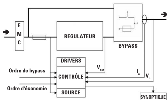
Fig. 9. Diagramme de blocs ILUEST+ .
