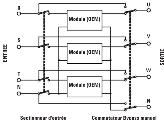
Fig. 11. Schéma connexion du Bypass manuel.
