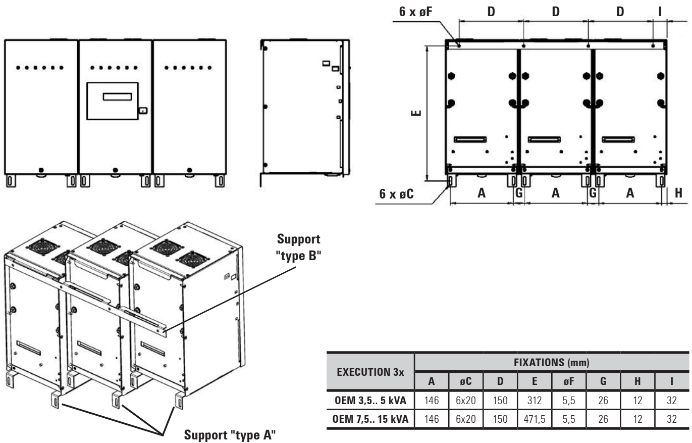
Fig. 15. Plan fixation système triphasé exécution (OEM).
