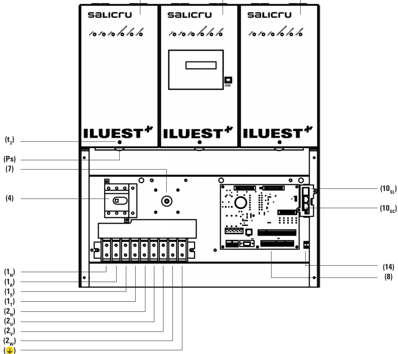
Détail agrandi de la vue frontale de l'ILUEST+ exécution dos de tableau (T) dans format horizontal et sans la couvercle de protection des bornes (Tb).
