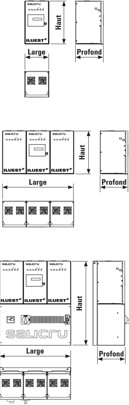
Fig. 31. Profil des différentes exécutions.
