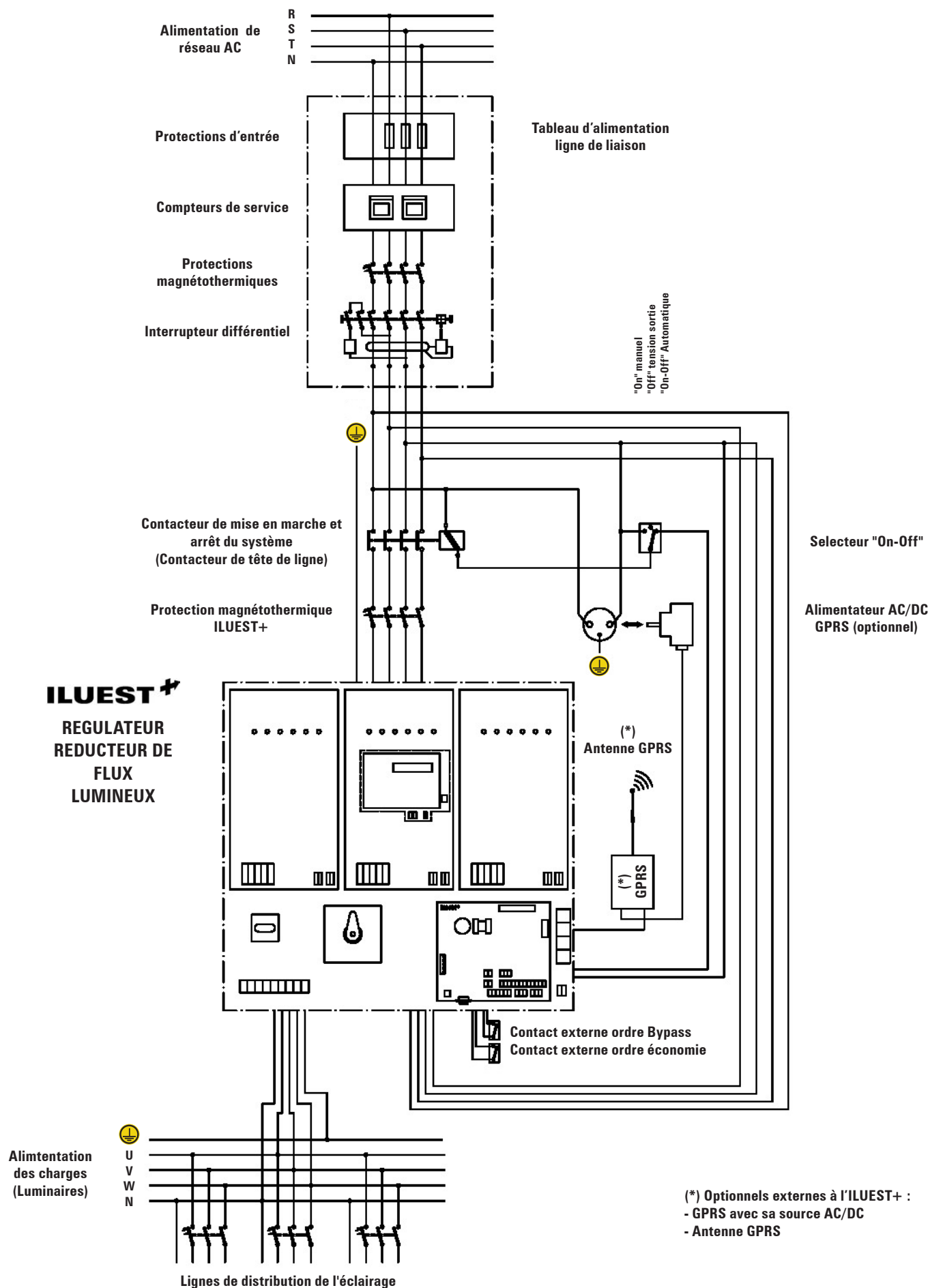
Fig. 18. Schéma connexion installation typique triphasée, appareil en exécution (T) ou (I) et avec carte concentratrice de base BM491*01.
