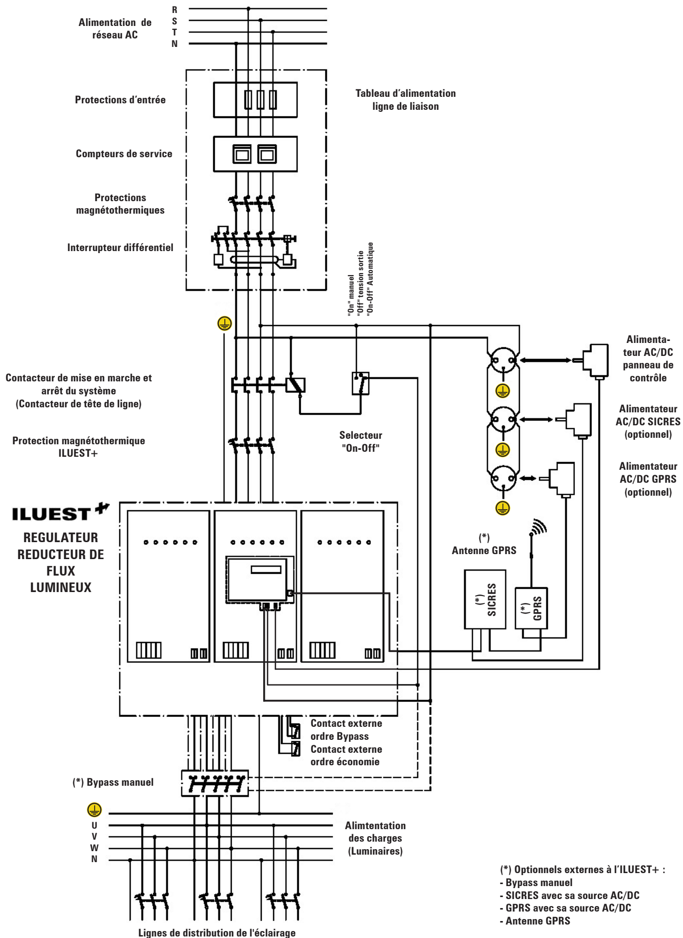
Fig. 17. Schéma connexion installation typique triphasée, appareil en exécution (OEM).
