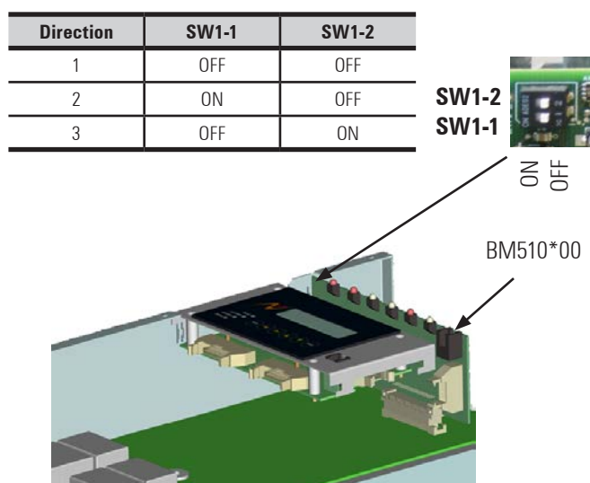
Fig. 30. Micro-switch SW1 réglage direction module.
