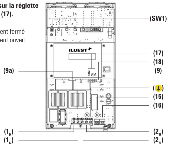
Module avec écran LCD dans format n° 1.
