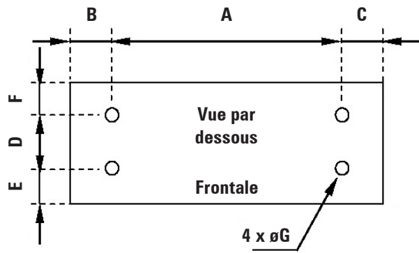
Plan fixation appareils en dos de tableau (T) et à l'intempérie (I).
