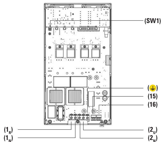
Module basique dans format n° 1.
