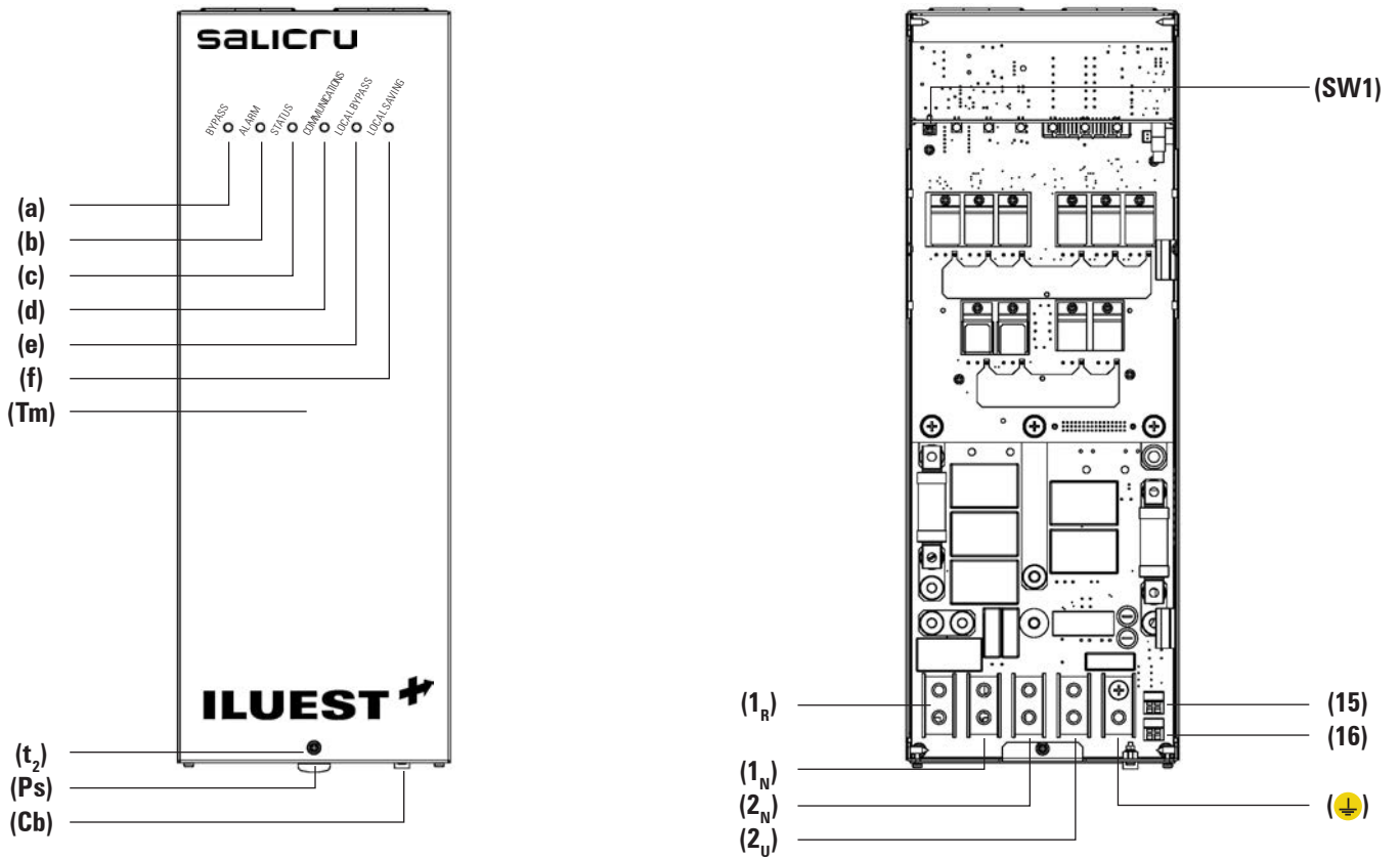
Module basique dans format n° 2.
