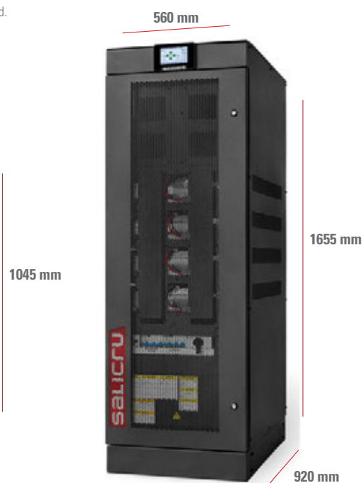
SLC-50÷80-CUBE4
