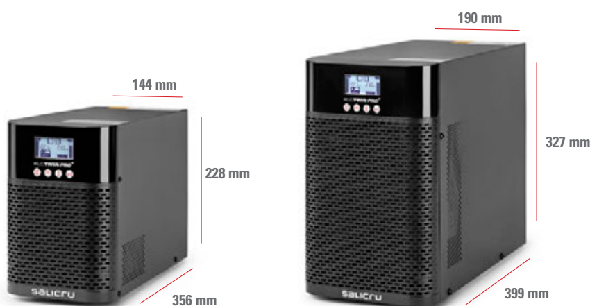
SLC 700/1000 TWIN PRO2 (IEC)
