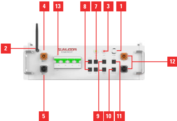
MODULE DE CONTRÔLE (BMS)
