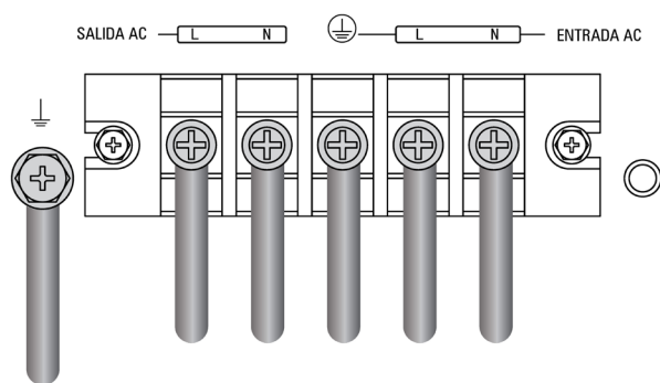
Fig. 39. Borneos E/S SLC TWIN PRO3.
