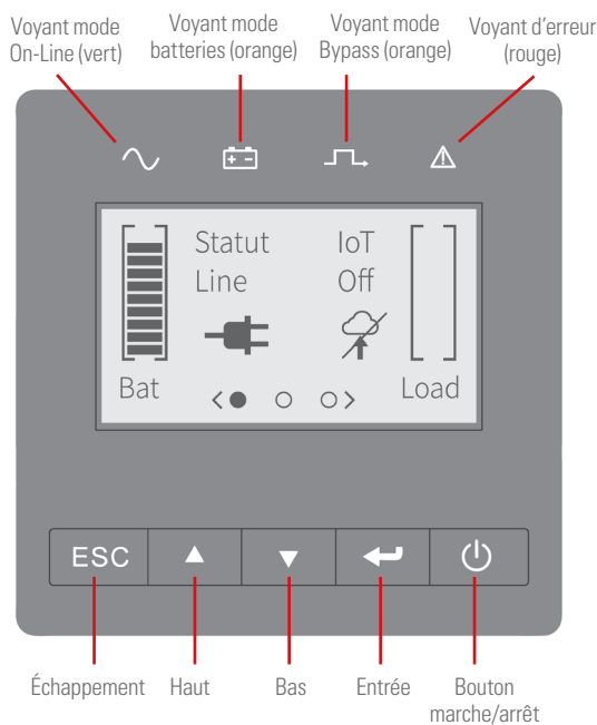
Fig. 59. Afficheur LCD.
