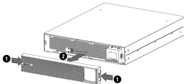
Fig. 26. Dépose de la façade.
