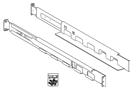
Fig. 13. Sliding guide kit.
