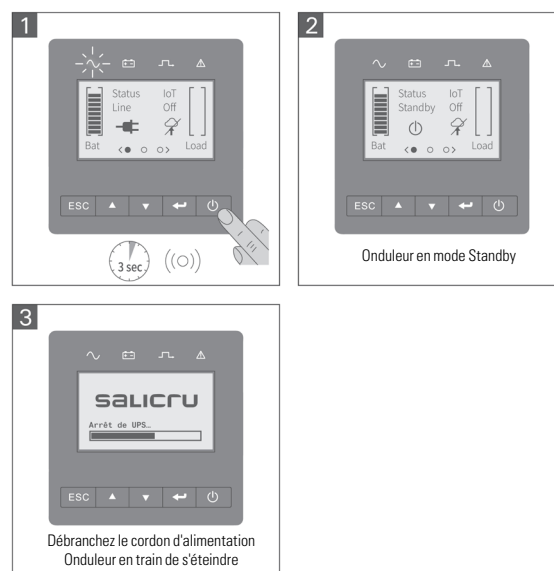
Fig. 58. Séquence d'arrêt.
