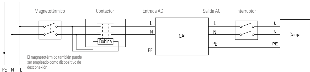
Fig. 36. Esquema de conexión E/S del SAI.
