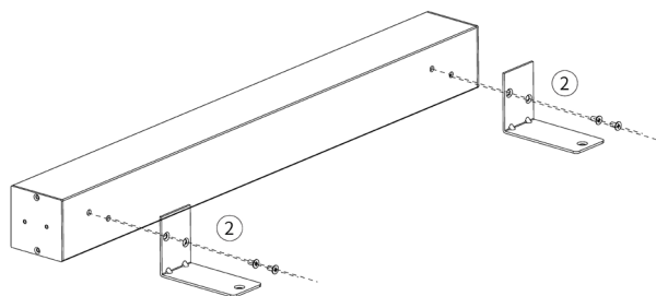
Fig. 34. Instalación de los soportes.
