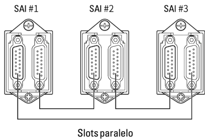
Fig. 49. Diagrama de conexión de la señal de paralelo.
