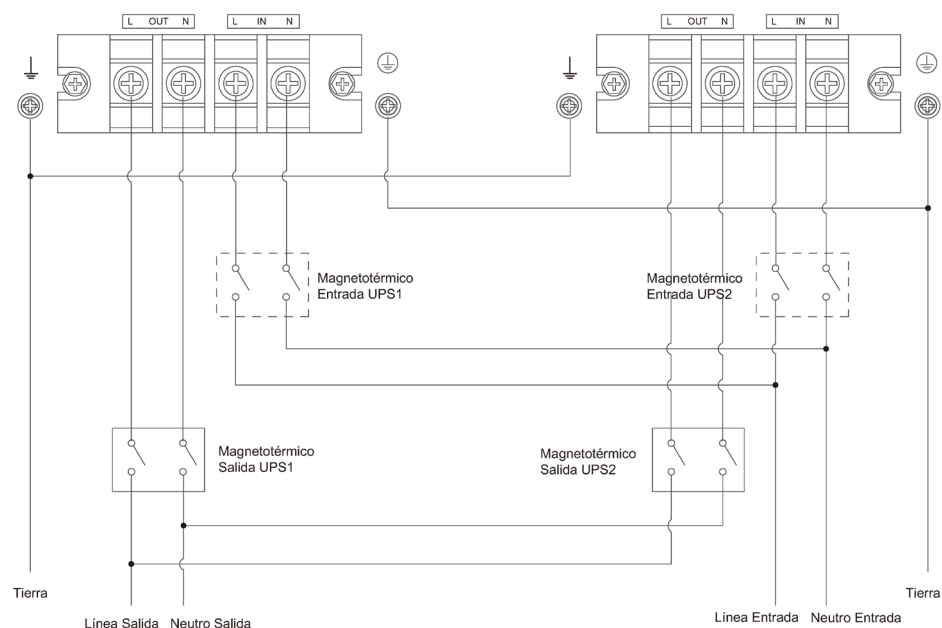
Fig. 48. Esquema cableado sistema paralelo SLC TWIN RT3.
