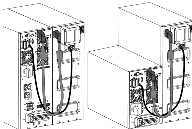
Fig. 41. Raccordement de l'onduleur SLC TWIN PRO3 à l'EBM.
