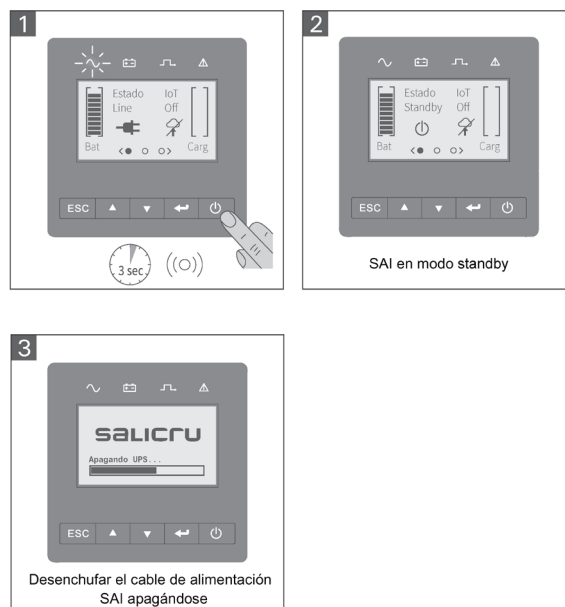
Fig. 58. Secuencia de apagado.
