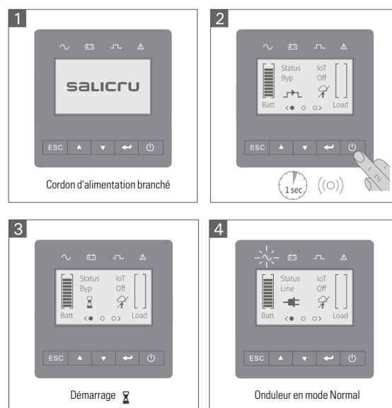
Fig. 56. Séquence de démarrage de l'onduleur.
