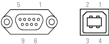
Fig. 51. Conectores DB9 para RS232 y USB.
