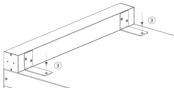
Fig. 35. Fijación de la PDU encima del SAI.
