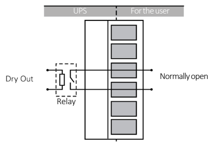
Fig. 54. Dry out diagram.
