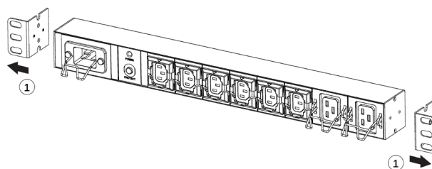
Fig. 33. Instalación de la PDU.
