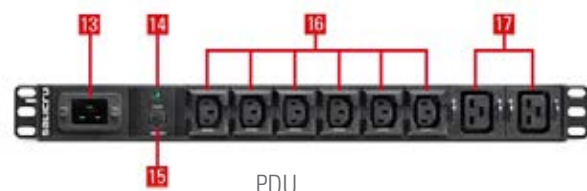
PDU
