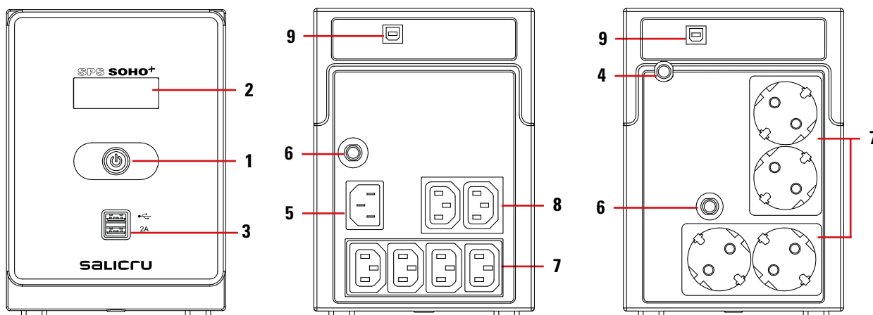
Fig. 2. Vue modèle SPS.SOHO+ 1 200 VA.
