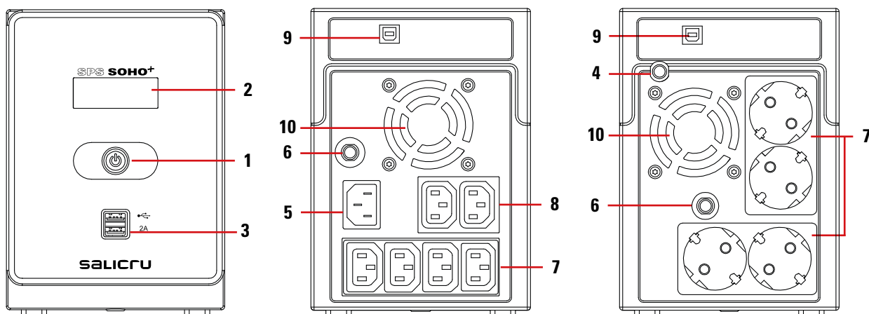
Fig. 3. Vue modèles SPS.SOHO+ 1 600 / 2 200 VA.
