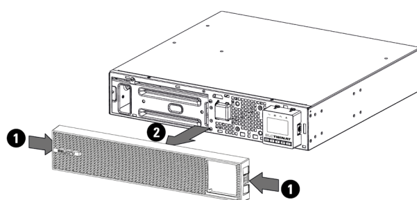
Fig. 15. Dépose de la façade.
