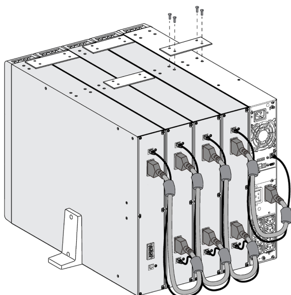
Fig. 21. União dos módulos diferentes.
