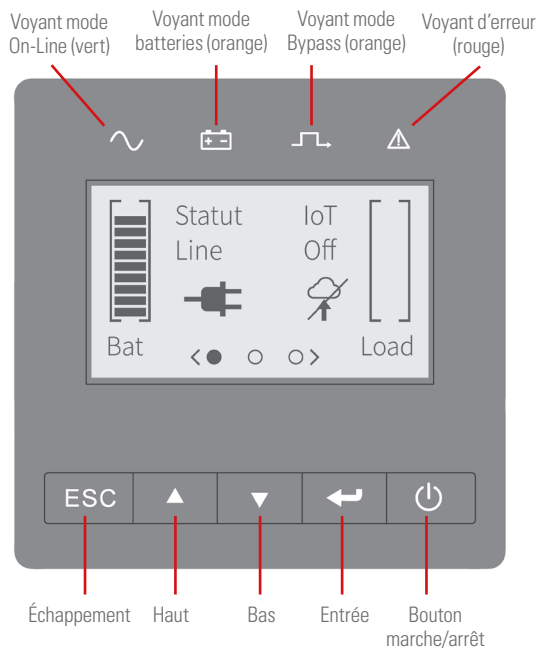
Fig. 31. Afficheur LCD.
