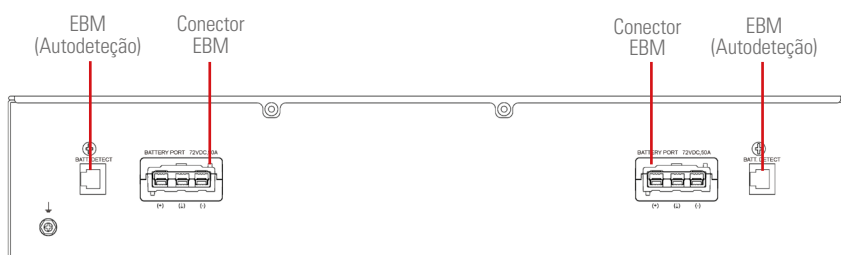
Fig. 6. Vista posterior módulo EBM de 72 V de baterias.
