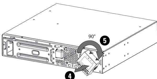
Fig. 17. Rotação do monitor LCD.
