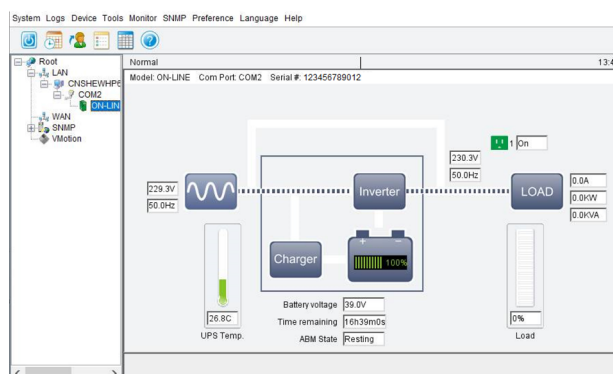
Fig. 26. Vue de l'écran principal du logiciel WinPower.
