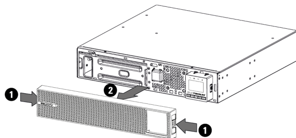
Fig. 15. Extração do painel frontal.
