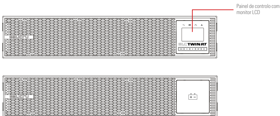
Fig. 1. Vista frontal modelos standard e B1 de 0,7 a 3 kVA (acima) e módulo EBM 36 V / 72 V de baterias para autonomias ampliadas (abaixo).
