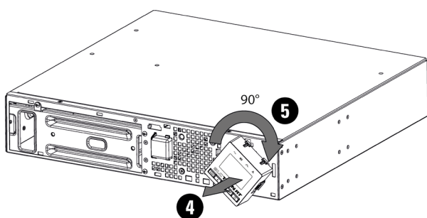
Fig. 17. Rotation de l'afficheur LCD.
