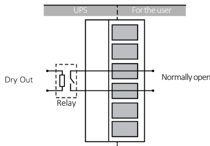
Fig. 25. Dry out diagram.
