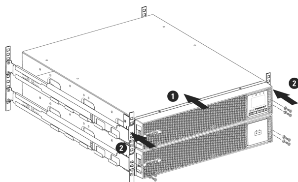
Fig. 14. Instalação do UPS com um módulo de baterias opcional.
