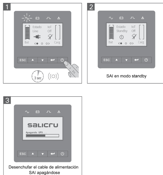
Fig. 30. Secuencia de apagado.
