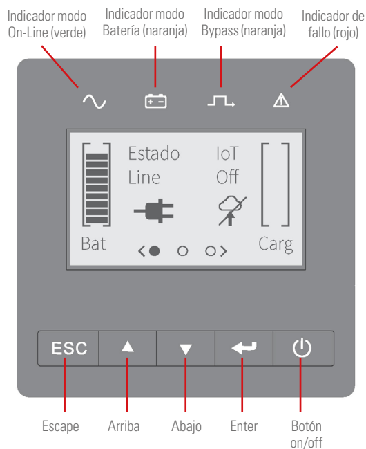
Fig. 31. Display LCD.
