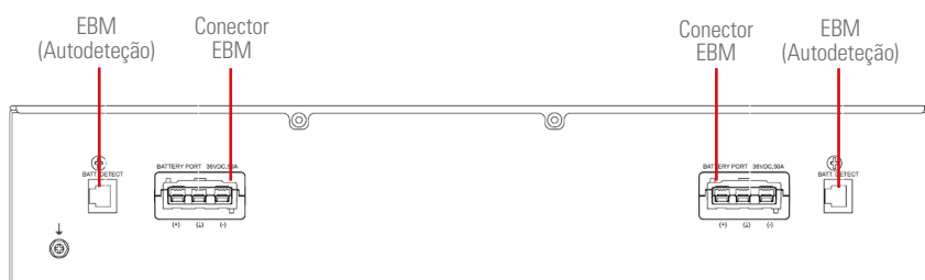
Fig. 5. Vista posterior módulo EBM de 36 V de baterias.
