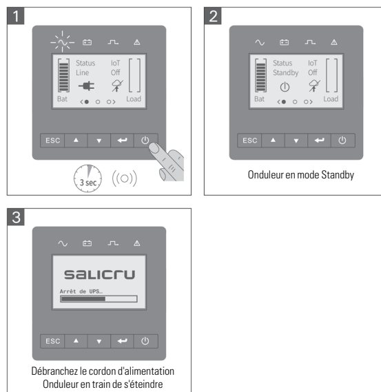
Fig. 30. Séquence d'arrêt.
