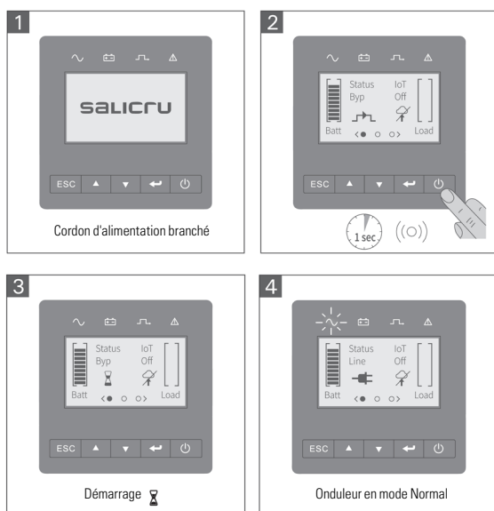
Fig. 28. Séquence de démarrage de l'onduleur.
