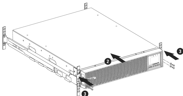
Fig. 13. Fijación del módulo SAI en el armario rack.
