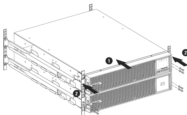
Fig. 14. Instalación del SAI con un módulo de baterías opcional.
