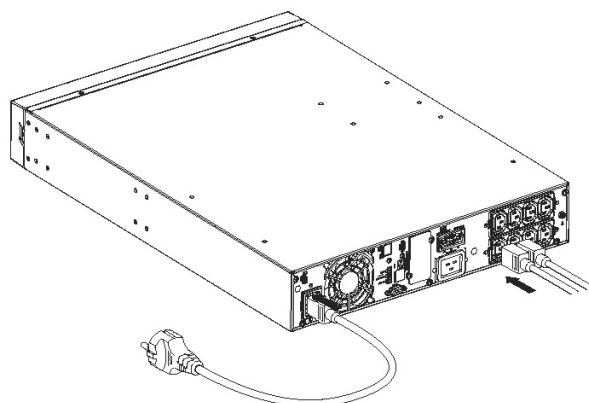
Fig. 19. Branchement du cordon d'alimentation et du câble des charges.
