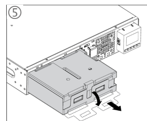
Fig. 42. Marche à suivre pour procéder au retrait des batteries internes.
