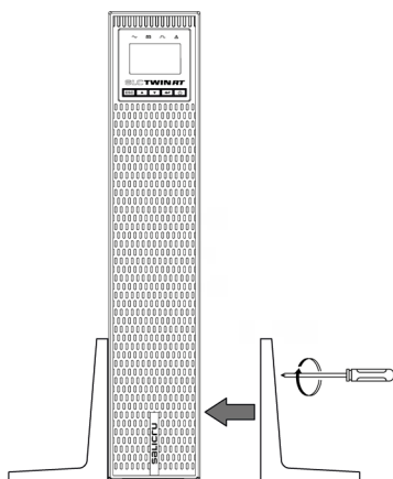
Fig. 18. Fijación de los soportes de instalación vertical.
