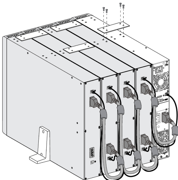
Fig. 21. Unión de los distintos módulos.
