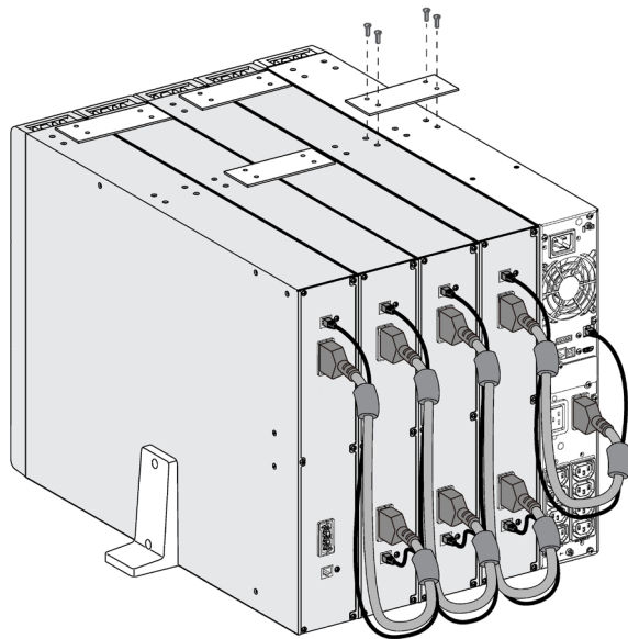
Fig. 21. Assemblage de plusieurs modules.
