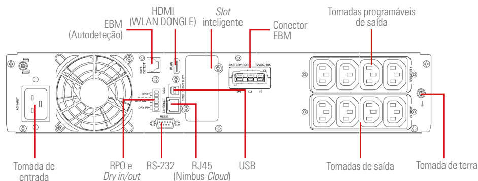
Fig. 3. Vista posterior modelo standard de 2 kVA.
