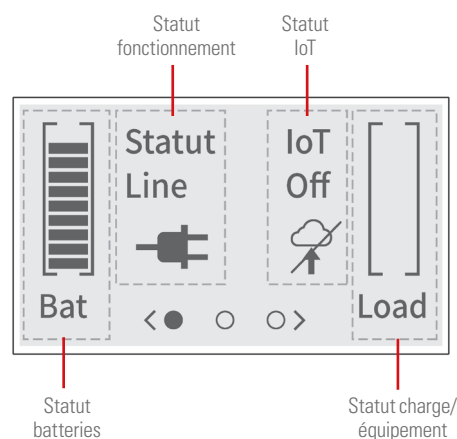
Fig. 34. Description de l'afficheur LCD.
