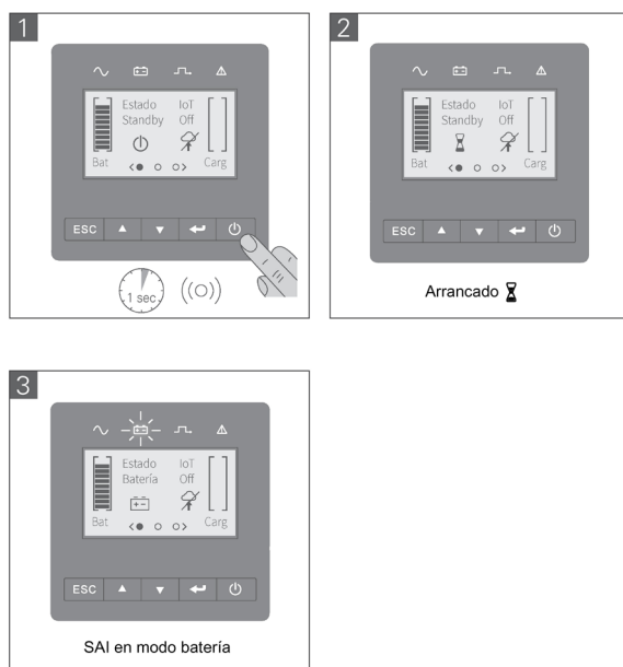
Fig. 29. Sequência de arranque a partir da bateria.
