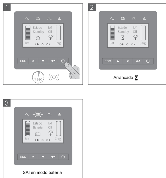
Fig. 29. Secuencia de arranque desde la batería.
