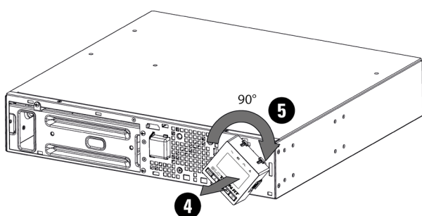
Fig. 17. Rotación del display LCD.
