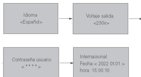
Fig. 27. Primeras pantallas de ajuste.
