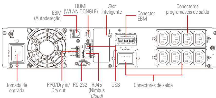
Fig. 4. Vista posterior modelos standard e B1 de 3 kVA.
