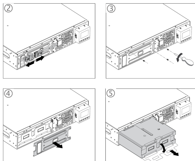
Fig. 42. Passos para a extração da bateria interna.
