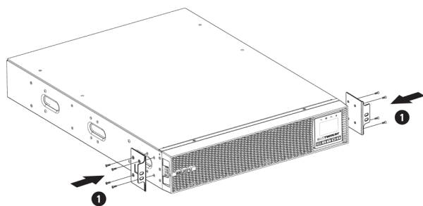
Fig. 12. Fixation des équerres de retenue.
