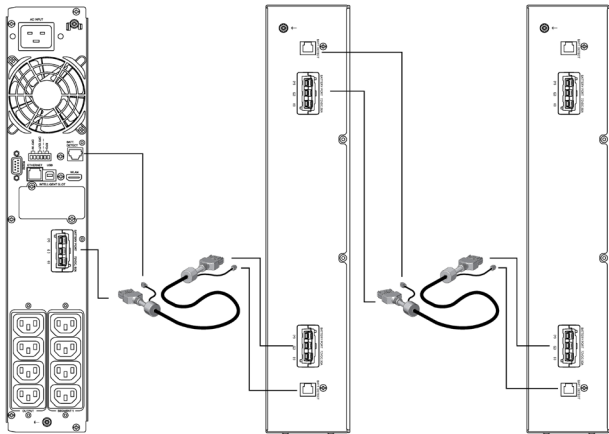
Fig. 20. Raccordement des modules de batteries à l'onduleur.
