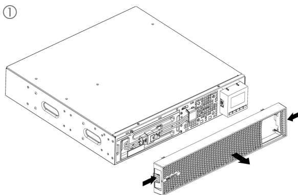
Fig. 41. Retrait de la façade.
