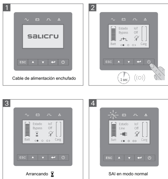
Fig. 28. Secuencia de arranque del SAI.
