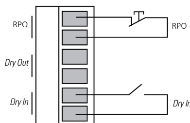
Fig. 24. Esquema de Dry in
