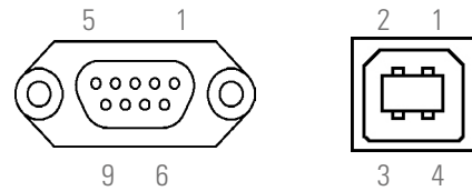
Fig. 22. Conectores DB9 para RS232 y USB.
