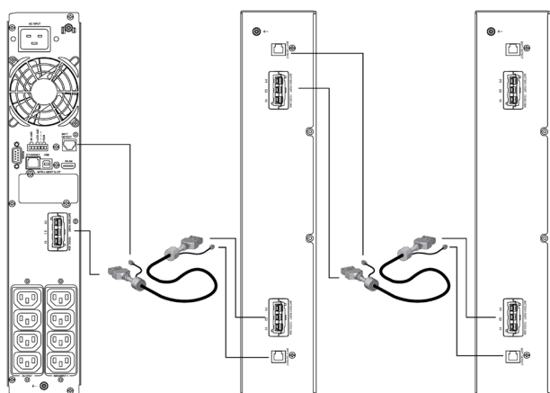
Fig. 20. Ligação dos módulos de bateria ao UPS.
