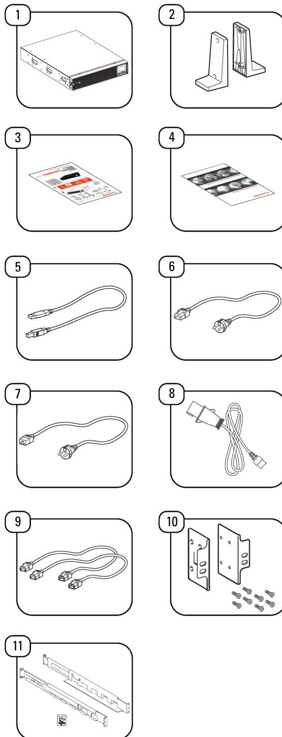
Fig. 10. Conteúdo da embalagem do UPS.
