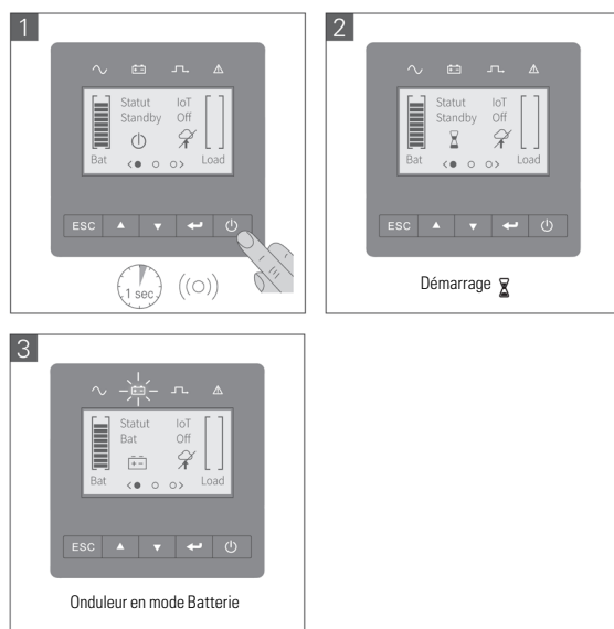
Fig. 29. Séquence de démarrage à partir des batteries.
