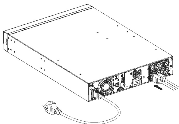
Fig. 19. Ligação do cabo de rede de entrada e cargas.
