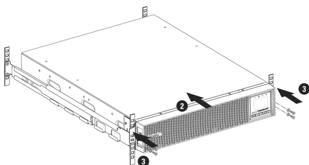
Fig. 13. Fixation du module ASI dans l'armoire rack.
