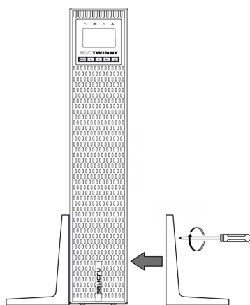
Fig. 18. Fixation des supports d'installation verticale.
