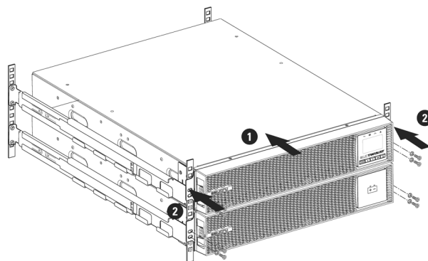
Fig. 14. Installation de l'onduleur avec un module de batteries en option.
