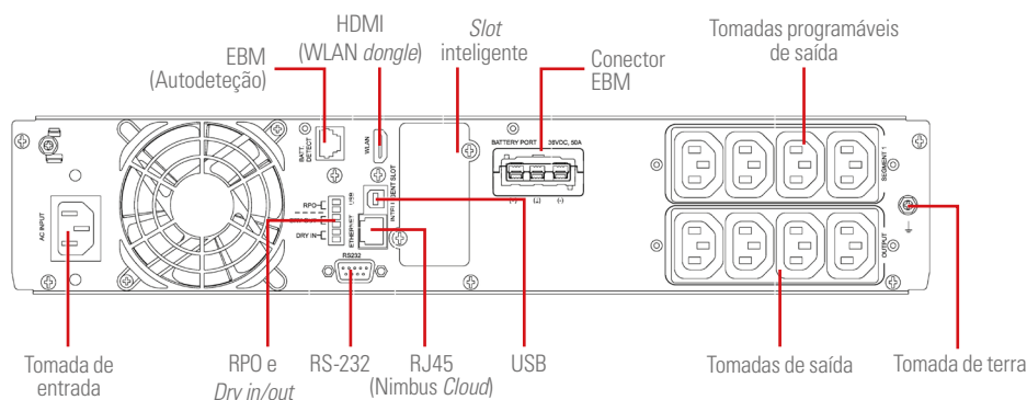
Fig. 2. Vista posterior modelos standard e B1 de 0,7 a 1,5 kVA.
