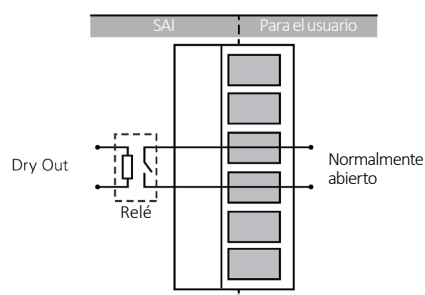
Fig. 25. Esquema Dry out.
