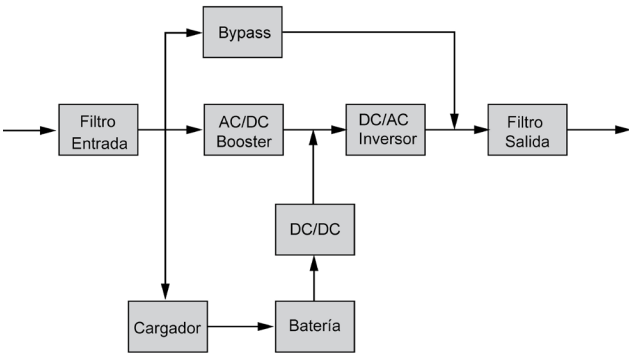
Fig. 7. Diagrama de blocos do UPS.
