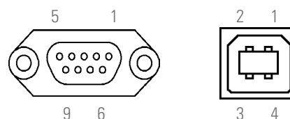
Fig. 22. Connecteurs DB9 pour RS-232 et USB
