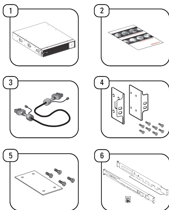
Fig. 11. Contenido del embalaje del módulo de baterías (EBM).
