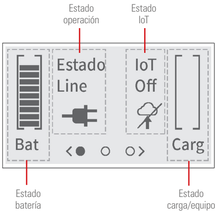
Fig. 34. Descripción del display LCD.
