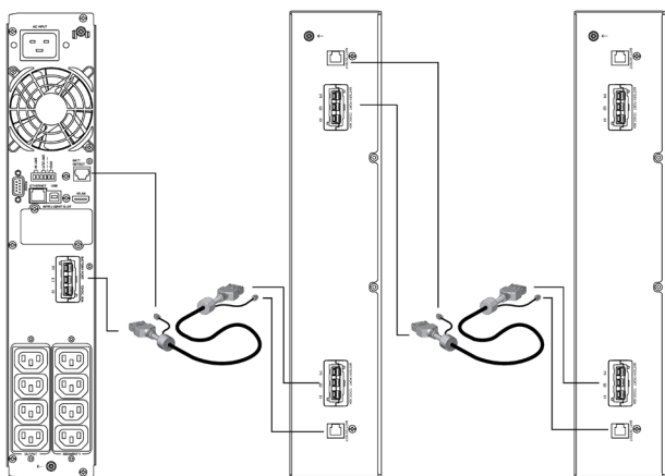
Fig. 20. Conexión de los módulos de batería al SAI.
