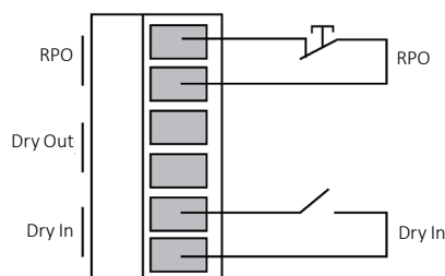
Fig. 24. Esquema Dry in
