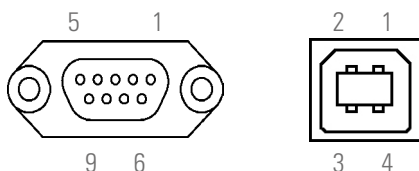
Fig. 22. Conectores DB9 para RS232 e USB.
