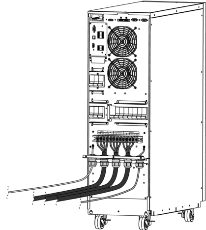
Fig. 36. Conexión configuración Entrada-Salida: trifásica-trifásica con línea de Bypass independiente en versión torre.
