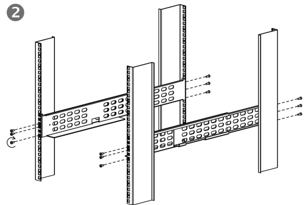
Fig. 47. Montaje de las guías en el armario rack.
