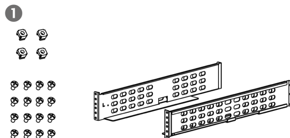
Fig. 46. Matériel nécessaire: guides et visserie.
