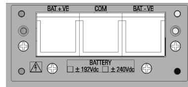
Détail B
