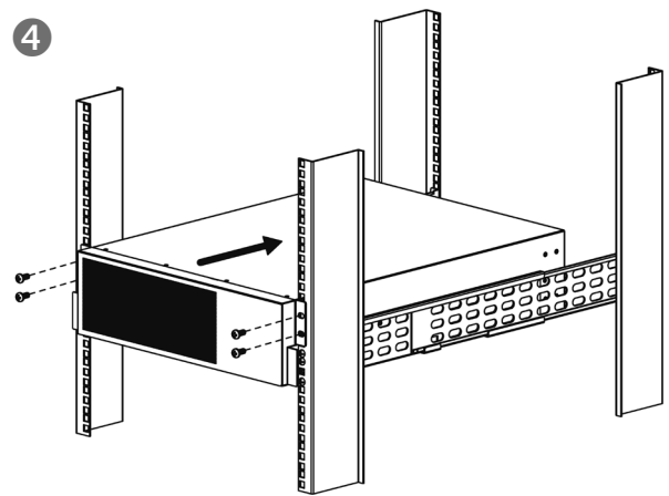
Fig. 53. Inserción y fijación de los módulos de batería en el armario rack.
