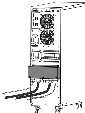
Fig. 41. Onduleur avec le couvercle de protection des terminaux de connexion en place en version tour.
