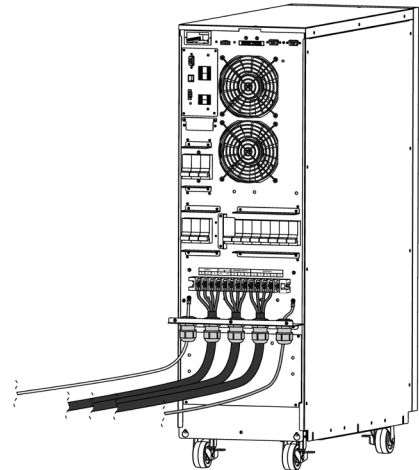
Fig. 36. Connexion de la configuration entrée-sortie : triphasée-triphasée avec ligne de bypass indépendant en version tour.
