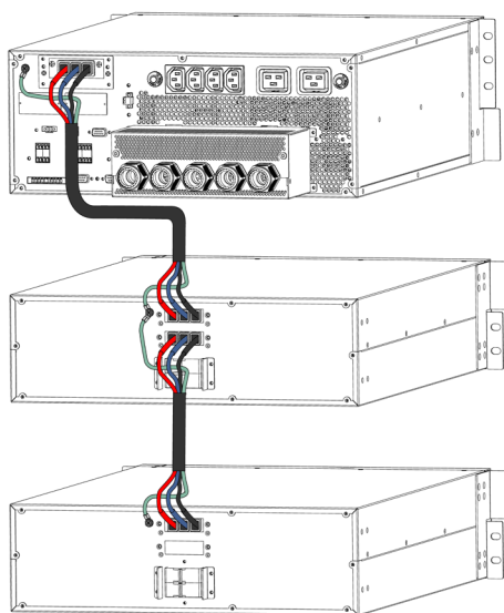
Fig. 44. Raccordement entre l'onduleur version rack 7,5 et 10 kVA et une ou plusieurs armoires batteries.
