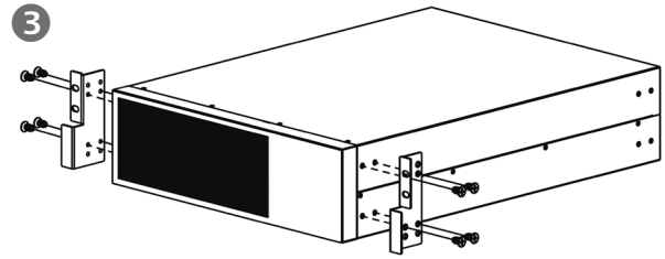
Fig. 52. Montage des supports dans les modules de batterie.
