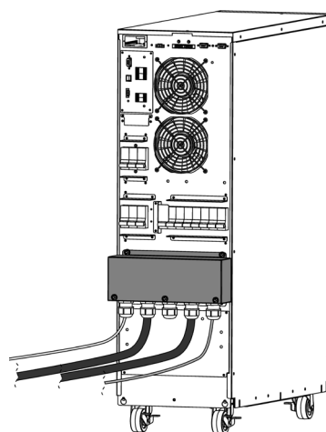
Fig. 41. SAI con la cubierta de protección de los terminales de conexión ubicada versión torre.
