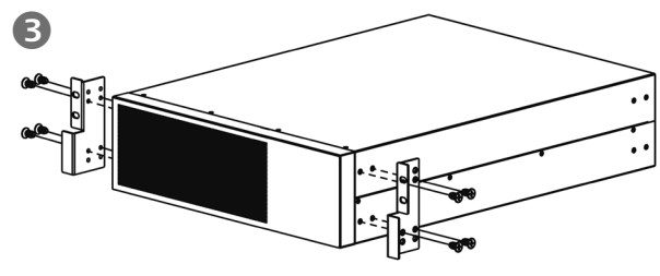
Fig. 52. Montaje de los soportes rack en los módulos de batería.
