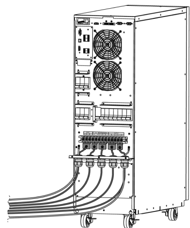
Entrada/Salida Monofásica-monofásica con línea de bypass independiente.
