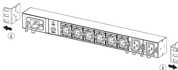
Fig. 32. Installation de la PDU.
