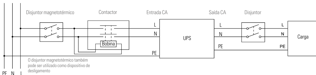
Fig. 35. Esquema de ligações E/S do UPS.
