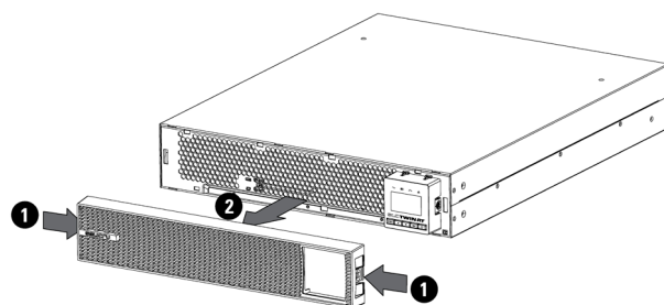
Fig. 25. Extracción del panel frontal.
