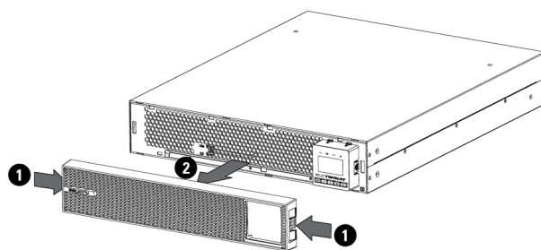
Fig. 25. Extração do painel frontal.
