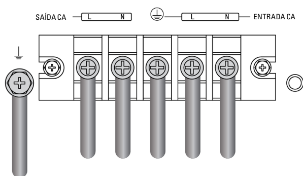
Fig. 38. Terminais E/S SLC TWIN PRO3.
