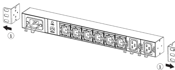
Fig. 32. Instalación de la PDU.
