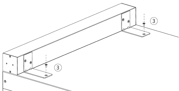
Fig. 34. Fixação da PDU sobre o UPS.
