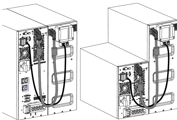
Fig. 40. Raccordement de l'onduleur SLC TWIN PR03 à l'EBM.
