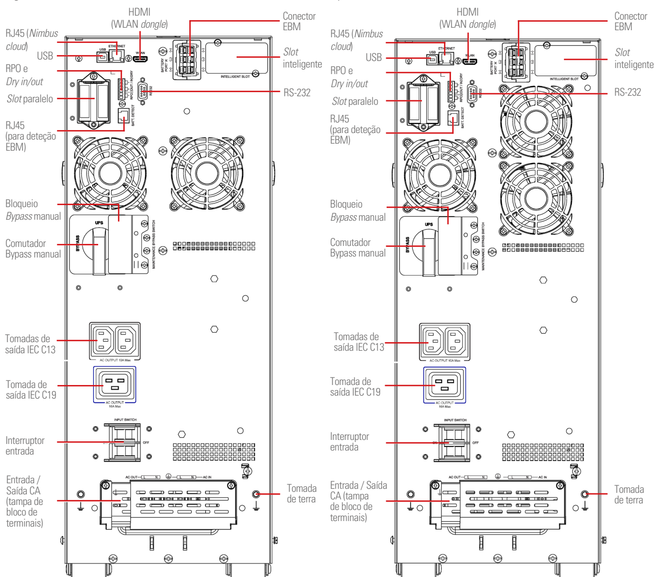
Fig. 3. Vista traseira da série SLC TWIN PRO3, modelos standard de 4/5/6 kVA (esq.) e 8/10 kVA (dir.).
