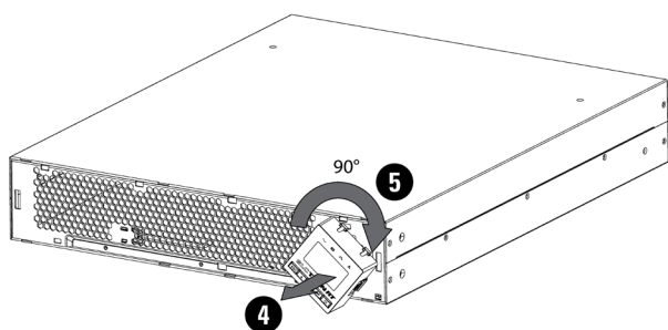
Fig. 27. Rotação do monitor LCD.
