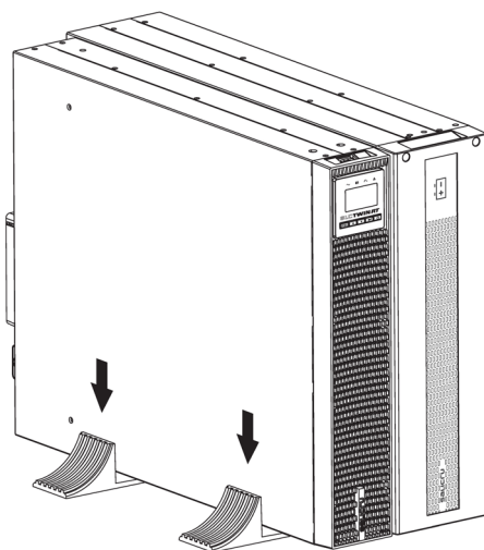
Fig. 31. Instalación del SAI + módulo de baterías en los soportes.
