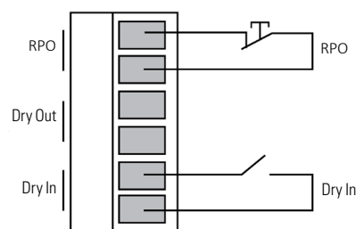
Fig. 51. Esquema de Dry in
