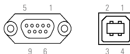
Fig. 50. Connecteurs DB9 pour RS-232 et USB.
