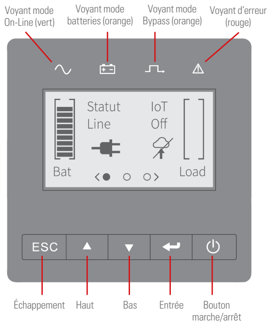
Fig. 57. Afficheur LCD.
