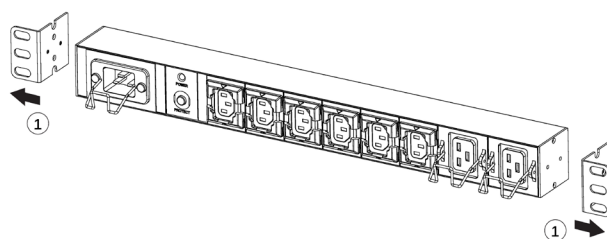
Fig. 32. Instalação da PDU.
