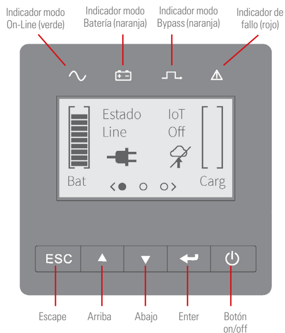
Fig. 57. Display LCD.
