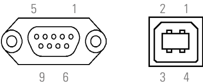
Fig. 50. Conectores DB9 para RS232 y USB.
