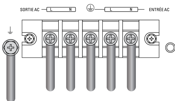
Fig. 38. Bornes entrée/sortie SLC TWIN PR03.
