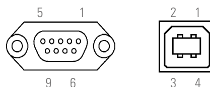
Fig. 50. Conectores DB9 para RS232 e USB.
