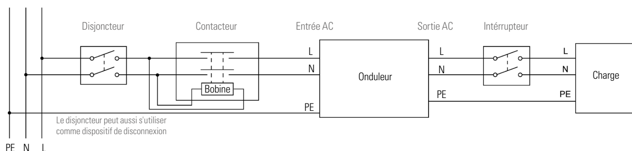
Fig. 35. Schéma de raccordement de l'entrée/sortie de l'onduleur.
