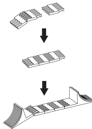
Fig. 30. Montaje de la platina de extensión.
