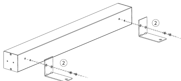
Fig. 33. Instalação dos suportes.
