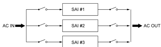
Fig. 45. Diagrama de ligação em paralelo.
