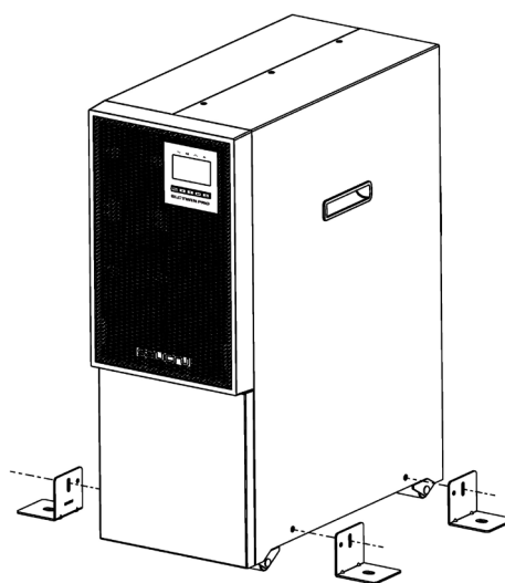
Fig. 21. Installation des supports de stabilisation.
