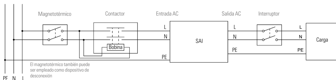
Fig. 35. Esquema de conexión E/S del SAI.
