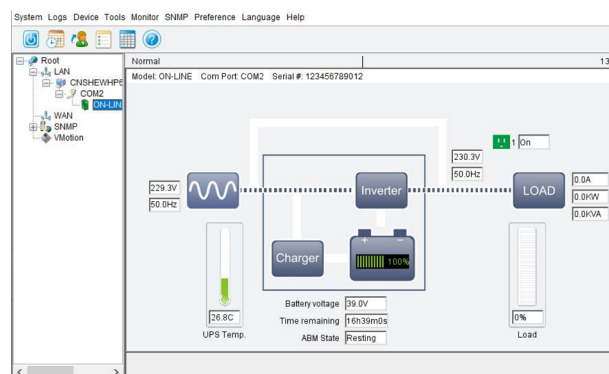
Fig. 53. Vue de l'écran principal du logiciel WinPower.
