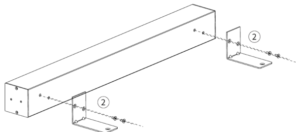
Fig. 33. Instalación de los soportes.
