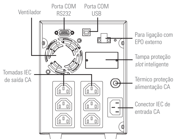
Vista posterior do equipamento standard .
