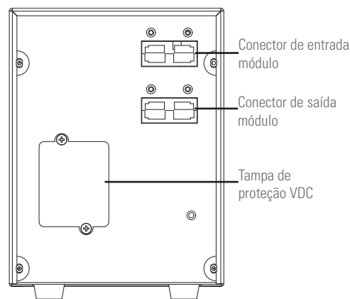
Vista posterior do módulo de baterias.
