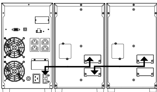
Fig. 8. Ligação com módulos de baterias.
