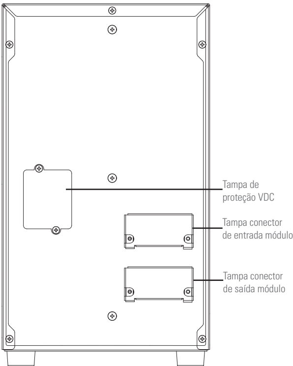
Vista posterior do módulo de baterias.
