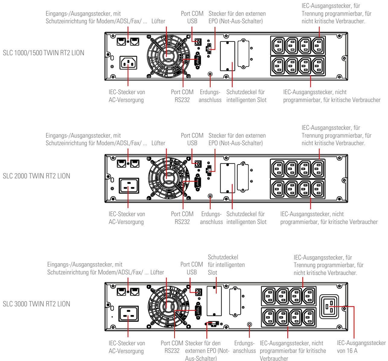
Abb. 2. Rückansicht der Modelle SLC TWIN RT2 LION.
