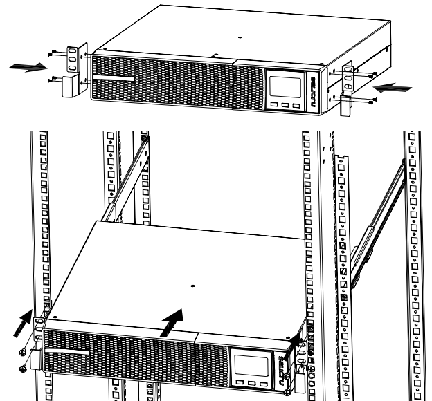
Abb. 5. Montage Typ Rack im 19"-Schrank.
