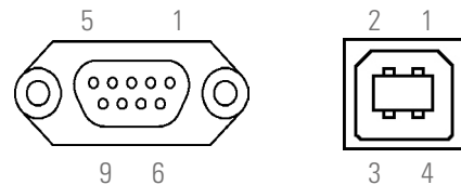
Abb. 7. Stecker DB9 für RS232 und USB.
