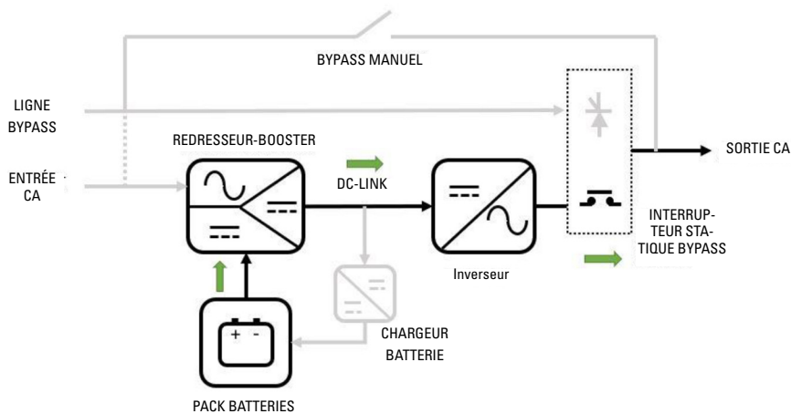
Fig. 15. Flux d'énergie de l'onduleur en mode batteries.
