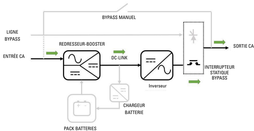
Fig. 19. Flux d'énergie de l'onduleur en mode convertisseur de fréquence.
