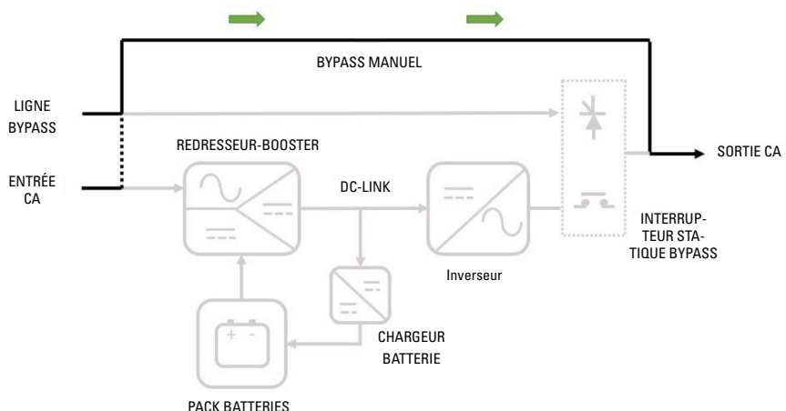
Fig. 17. Flux d'énergie de l'onduleur en mode bypass de maintenance.
