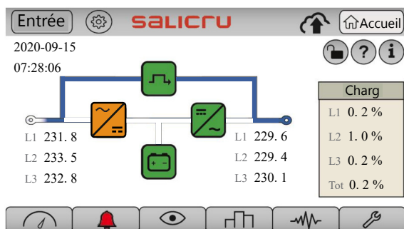
Fig. 54. Écran principal en mode bypass. Le flux d'énergie passe de l'entrée de bypass à la sortie directement, à travers l'interrupteur statique de bypass. Le redresseur et le chargeur restent en fonctionnement.
