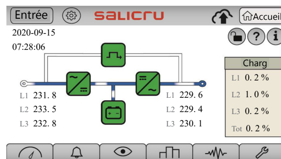
Fig. 52. Écran principal en fonctionnement normal. Le flux d'énergie doit correspondre à ce qui est affiché : l'entrée alimente le redresseur ; celui-ci alimente simultanément l'inverseur et le chargeur de batteries ; l'inverseur fournit l'énergie aux charges de sortie.
