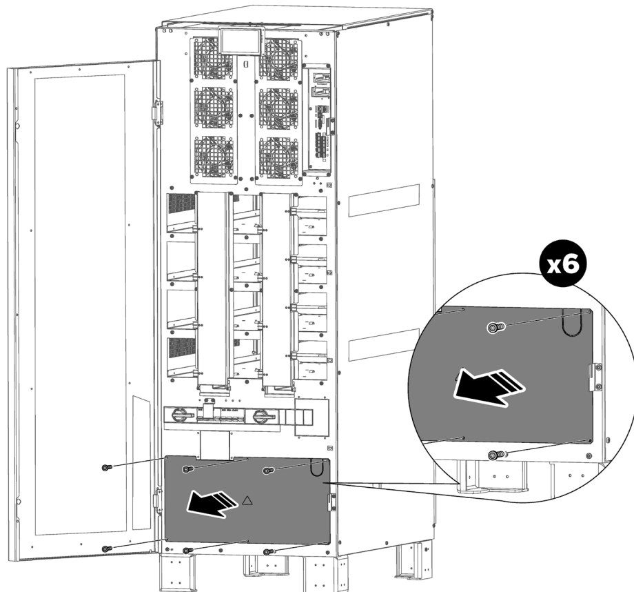
Fig. 43. Détail de la dépose du cache-bornes avant.
