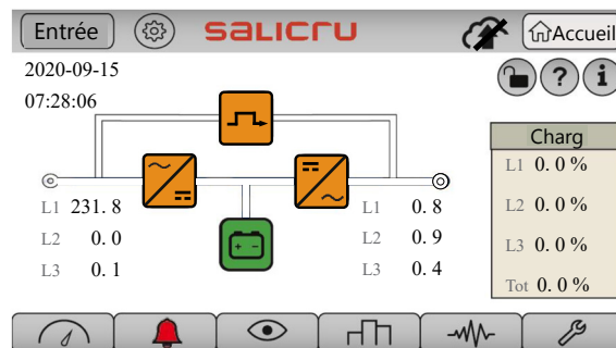
Fig. 61. Écran principal avec arrêt d'urgence EPO activé. Aucun flux d'énergie n'est représenté, il n'y a pas de tension de sortie.
