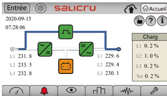
Fig. 56. Écran principal avec l'onduleur arrêté. Le flux d'énergie passe de l'entrée de bypass à la sortie directement, à travers l'interrupteur statique de bypass, et tous les convertisseurs sont arrêtés.
