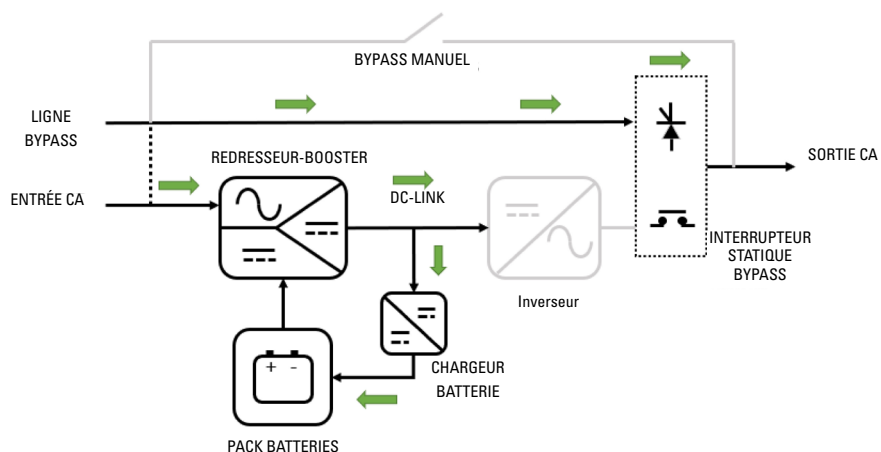
Fig. 18. Flux d'énergie de l'onduleur en mode ECO.
