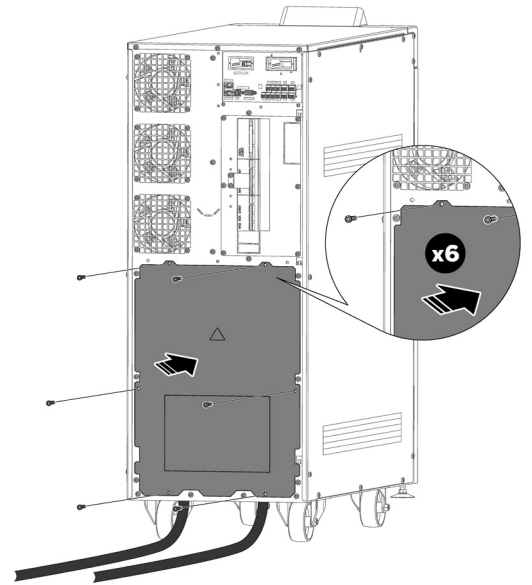
Fig. 42. Détail du repositionnement du cache-bornes arrière.
