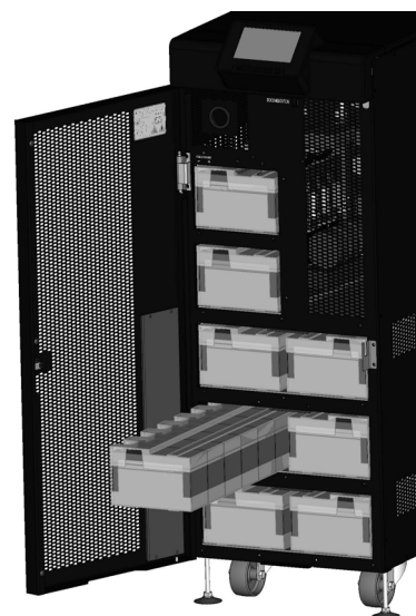
Fig. 38. Détail de l'accès avant aux batteries. Exemple équipements de 30 kVA et 40 kVA.
