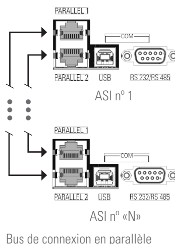
Fig. 49. Connecteurs RJ45 du bus de communication parallèle.
