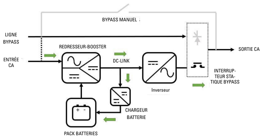
Fig. 14. Flux d'énergie de l'onduleur en mode normal.
