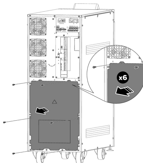
Fig. 39. Détail de la dépose du cache-bornes arrière.
