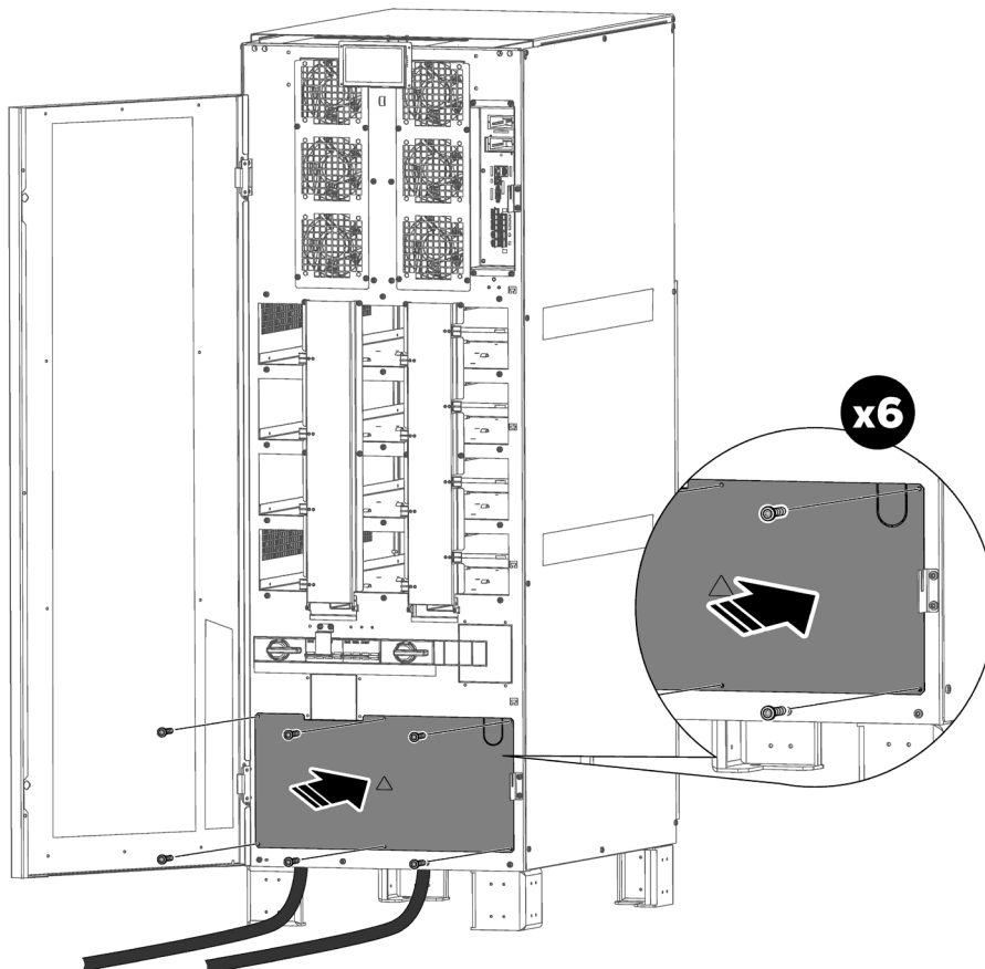
Fig. 46. Détail du repositionnement du cache-bornes avant.
