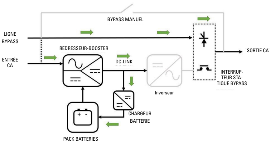
Fig. 16. Flux d'énergie de l'onduleur en mode bypass.
