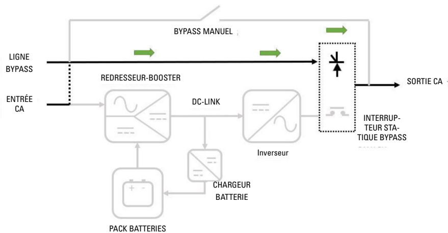
Fig. 13. Flux d'énergie de l'onduleur arrêté (mais alimentant les charges à travers le bypass).
