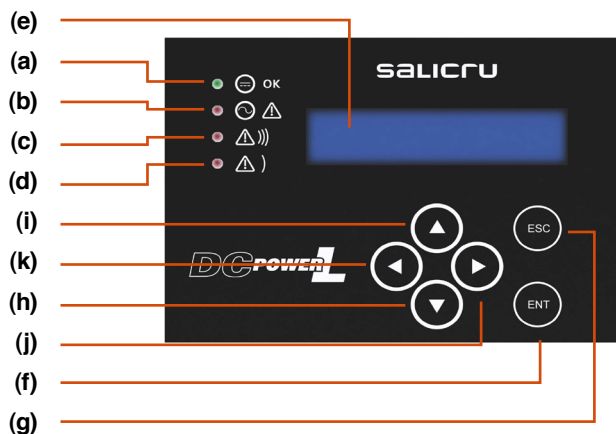
Fig. 1. Vista panel de control.
