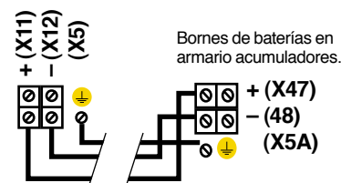
Fig. 15. Conexión sistema con un armario de baterías.
