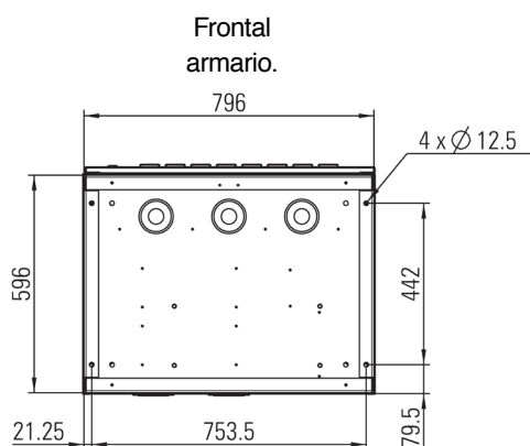
Armario con base 600x800.
