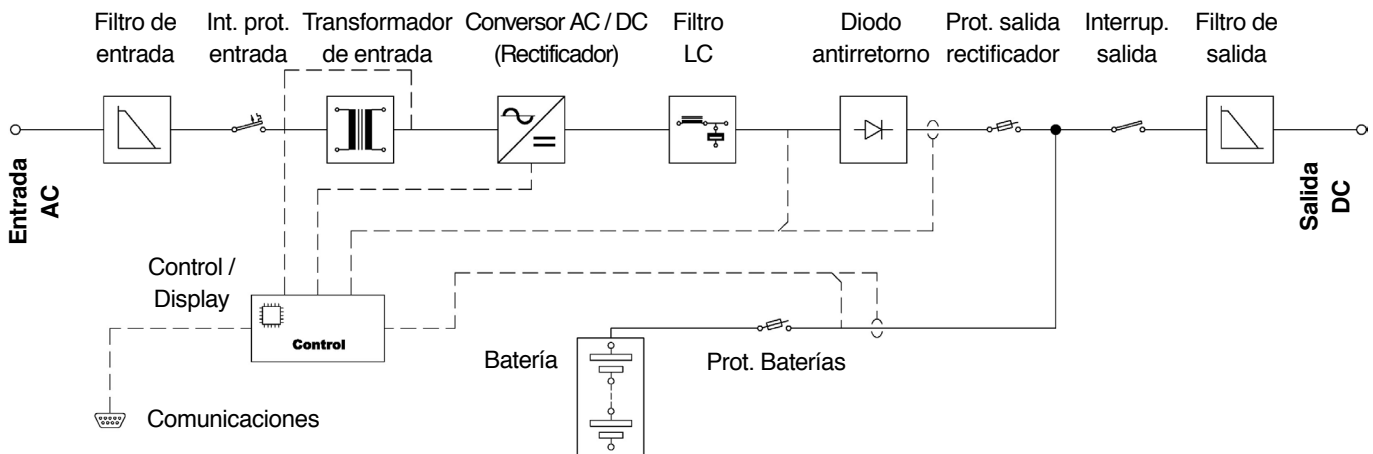
Fig. 12. Esquema de bloques.
