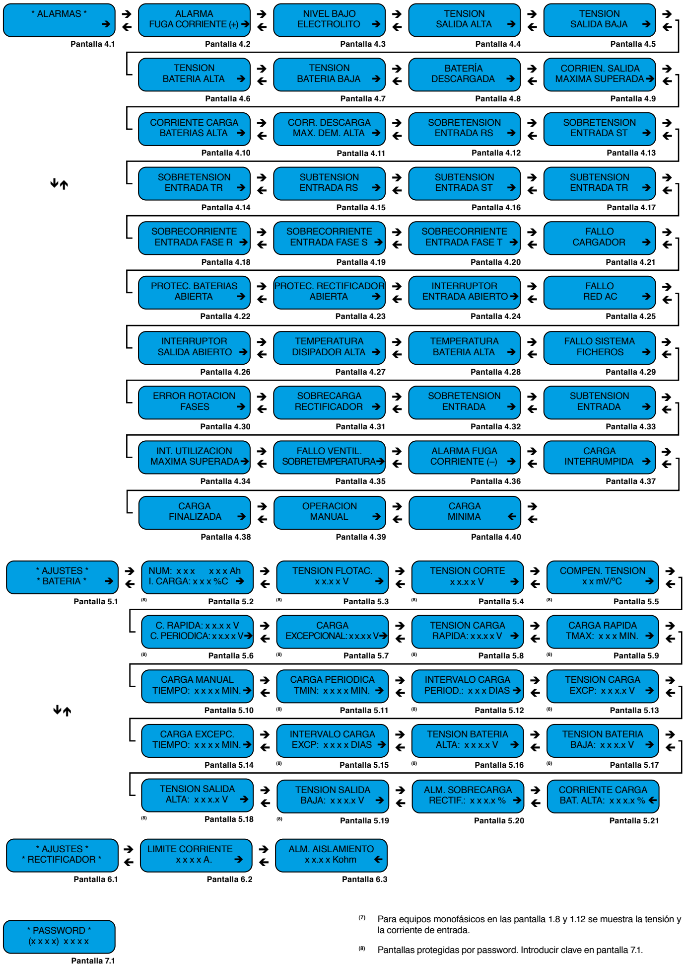
Fig. 19. Mapa de pantallas del panel de control.
