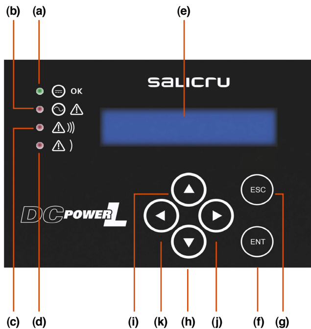
Fig. 18. Panel de control con display LCD.
