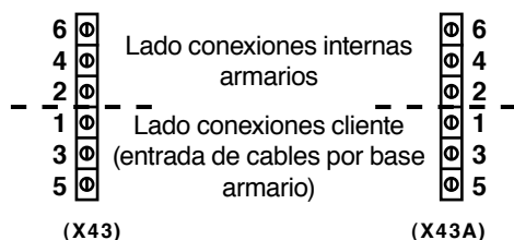
Armario rectificador
