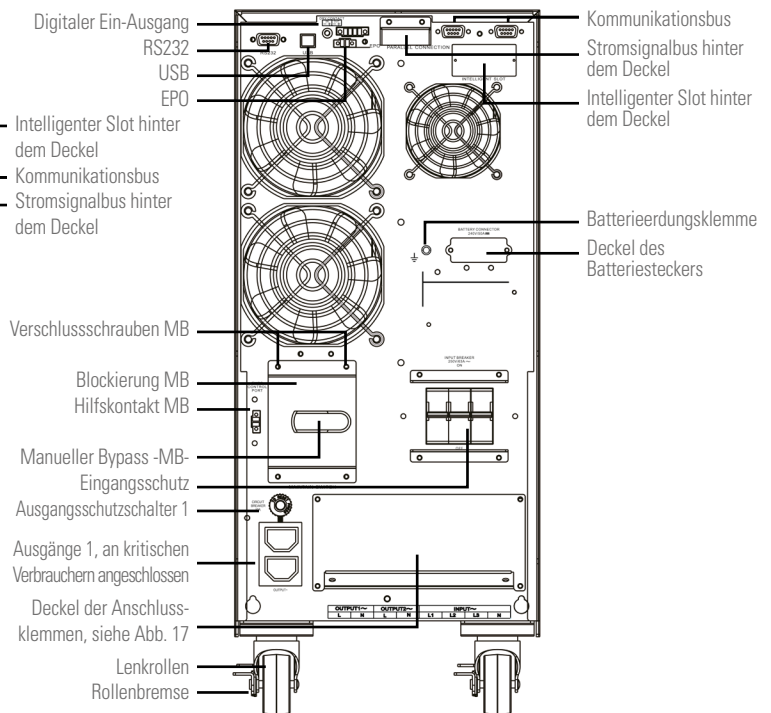
Von 8 bis 10 kVA Standard und B1. Dreiphasiger Eingang und einphasiger Ausgang.
