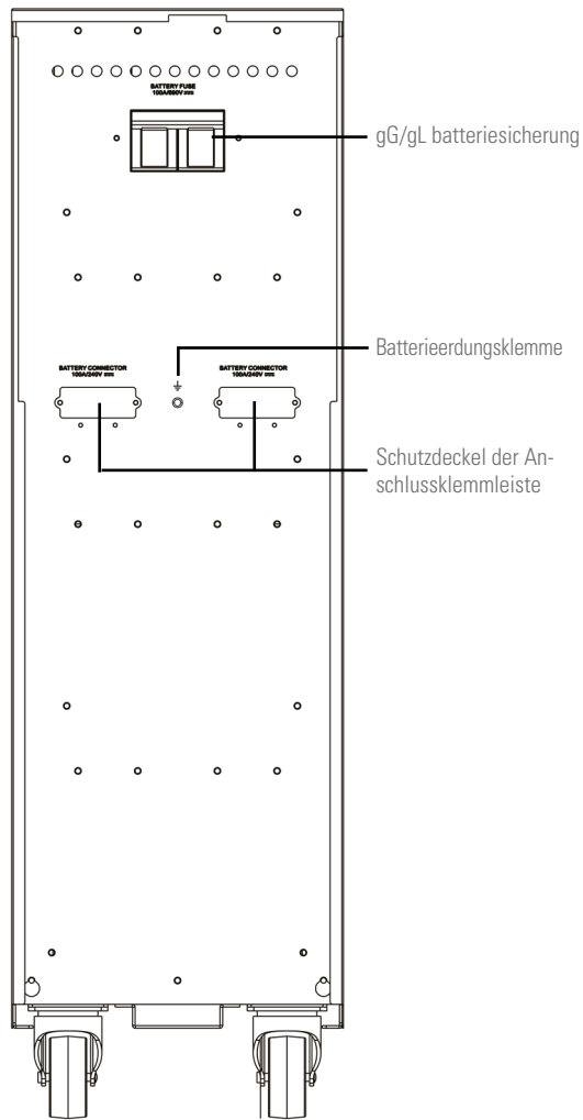
Batteriemodul Größe 2, mit 4x20 Elementen und Schutz von 100 A.
