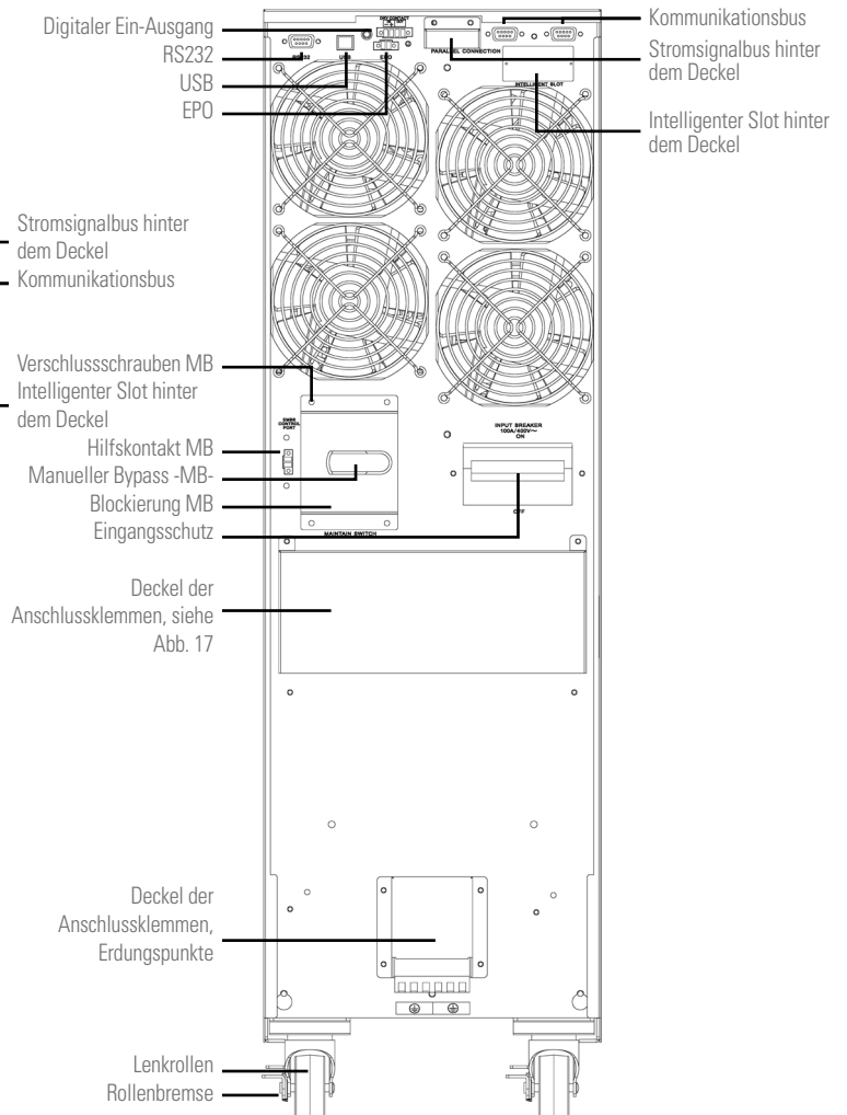
Von 15 und 20 kVA Standard. Dreiphasiger Eingang und einphasiger Ausgang.
