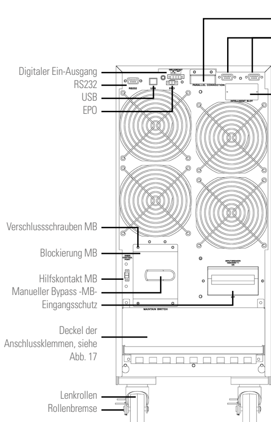
Von 15 und 20 kVA B1. Dreiphasiger Eingang und einphasiger Ausgang.
