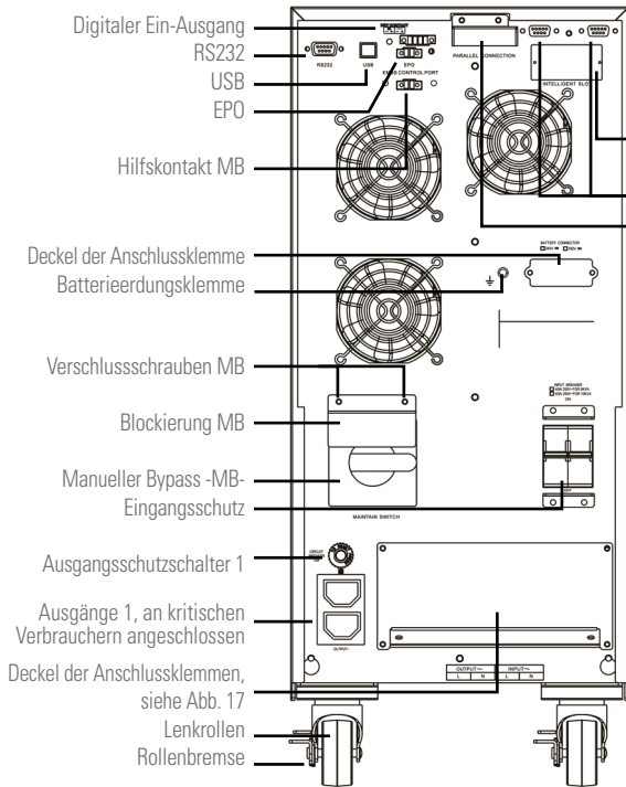
Von 4 bis 10 kVA Standard und B1. Einphasiger Eingang und Ausgang.
