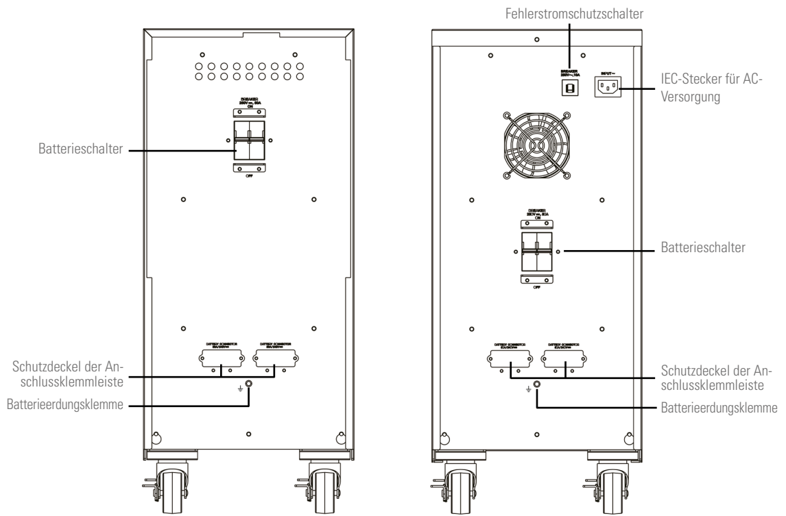
Batteriemodul Größe 1, mit 2x20 Elementen und Schutz von 50 A.
