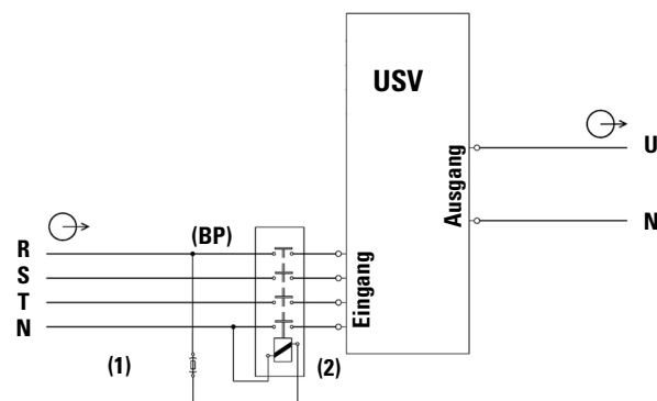
Anschluss „Backfeed protection“ für TWIN/3 PRO2.
