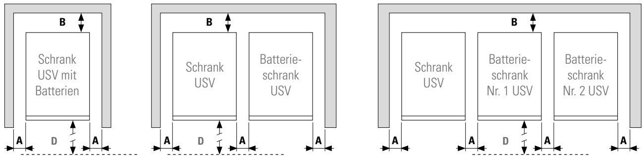
Abb. 14. Minimale Außenmaße für die Lüftung der USV.
