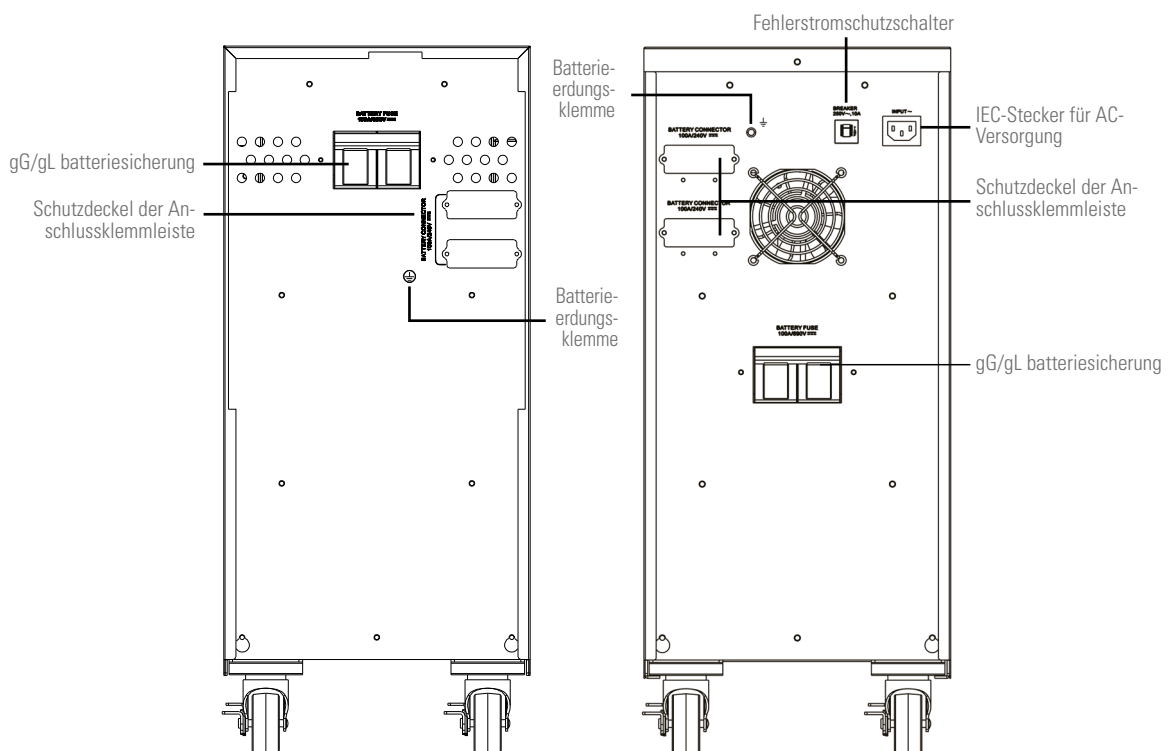
Batteriemodul Größe 1, mit 2x20 Elementen und Schutz von 100 A.
