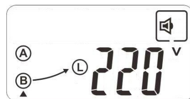
Abb. 10. Übertragungsbildschirm über den Eingang B.
