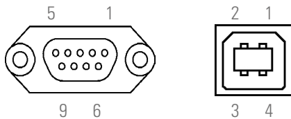
Abb. 5. DB9-Stecker für RS232 und Schnittstellenrelais und USB-Stecker.
