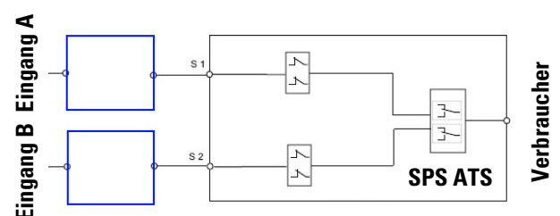
Abb. 3. Strukturelles Blockschema.
