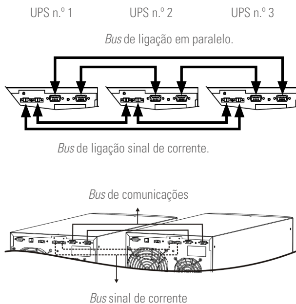
Fig. 22. Ligação bus de comunicação e sinal de corrente.
