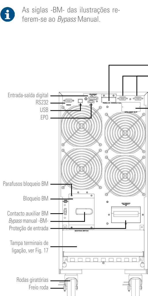
Fig. 2. Vista posterior modelos de 4 kVA a 20 kVA.
