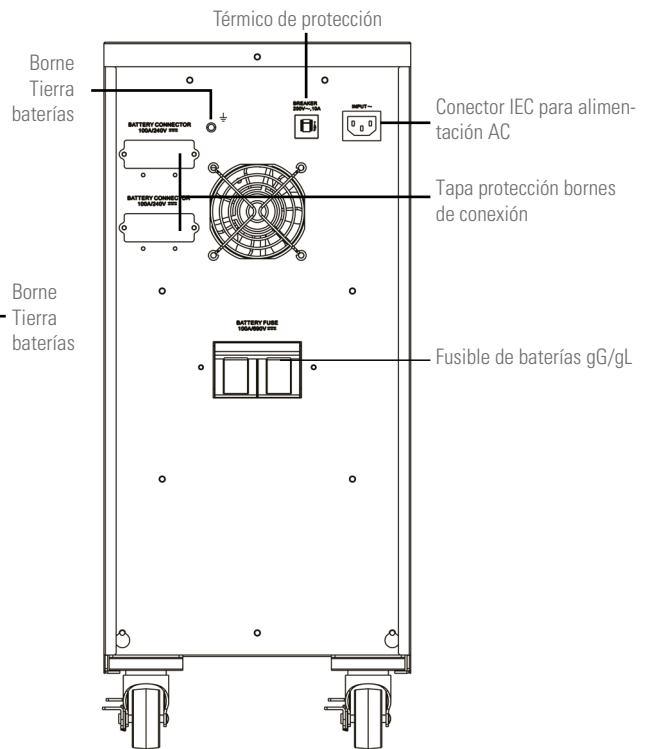
Módulo de baterías tamaño 1, con 3x20 elementos y protección de 100 A.
