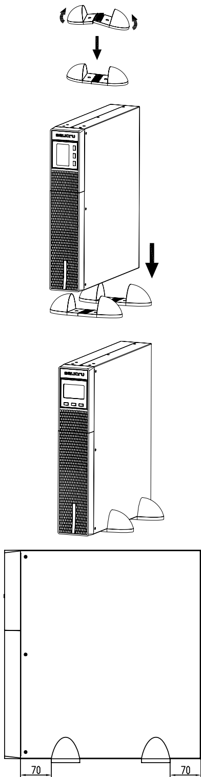
Fig. 6. Montaje vertical -tipo torre-.
