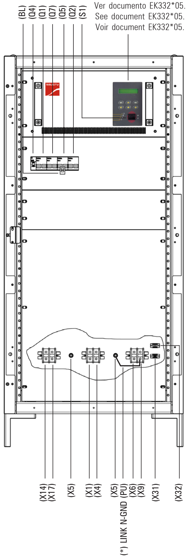
Fig. 8. Vista frontal ONDULADOR en armario. Front view of the INVERTER in cabinet. Vue frontale CONVERTISSEUR en armoire.
