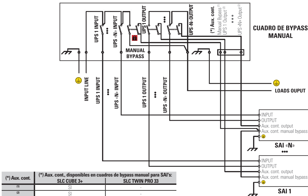
Fig. 5. Cuadro de bypass manual para «n» SAI's estándar en paralelo o redundante, de la serie CUBE3+ y TWIN PRO 33.
