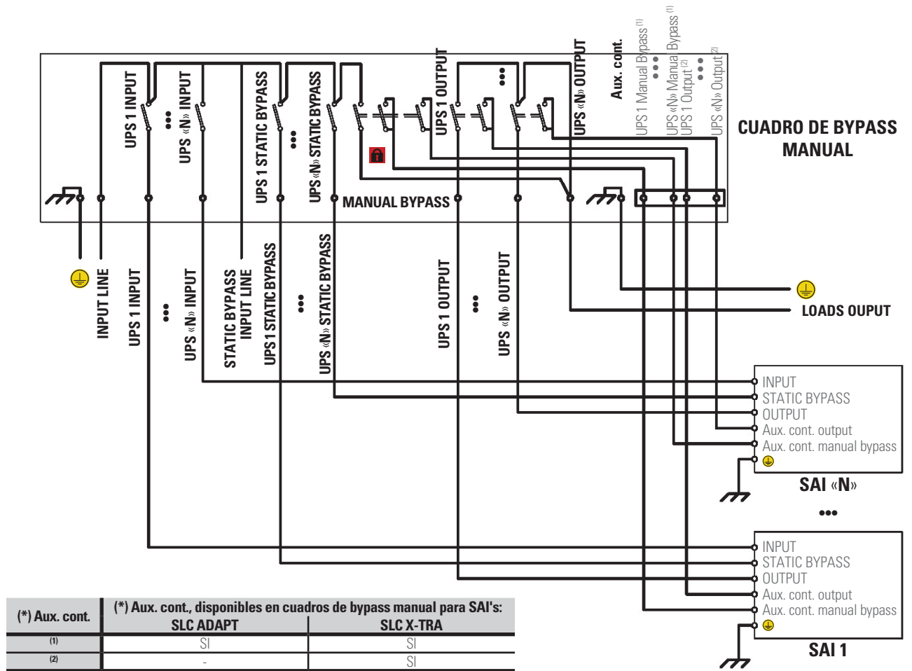
Fig. 8. Cuadro de bypass manual para «n» SAI's con línea de bypass independiente en paralelo o redundante, de la serie ADAPT y X-TRA.
