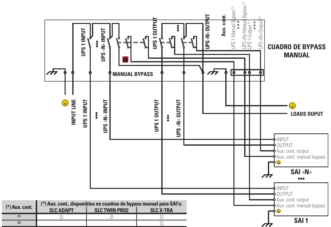
Fig. 6. Cuadro de bypass manual para «n» SAI's estándar en paralelo o redundante, de la serie ADAPT, TWIN PRO2 y X-TRA.
