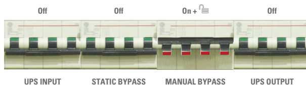
Fig. 13. Posición de los interruptores del cuadro de bypass en «Funcionamiento de mantenimiento» (con un SAI).
