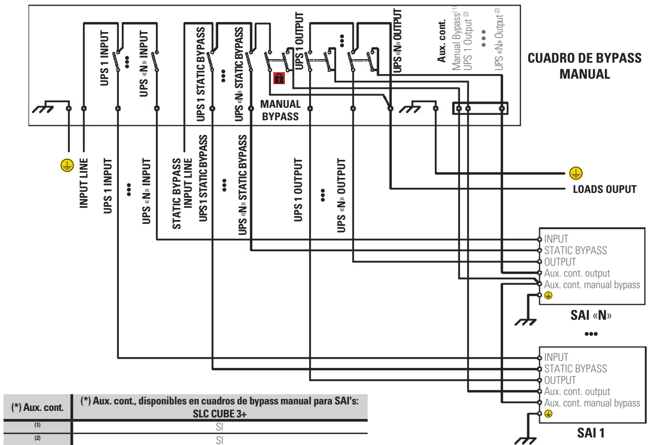
Fig. 7. Cuadro de bypass manual para «n» SAI's con línea de bypass independiente en paralelo o redundante, de la serie CUBE3+.
