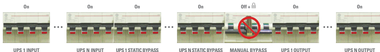
Fig. 12. Posición de los interruptores del cuadro de bypass en «Funcionamiento normal» (con varios SAI's).
