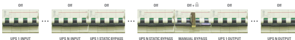
Fig. 10. Posición de los interruptores del cuadro de bypass en «Fuera de servicio» (con varios SAI's).
