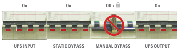
Fig. 15. Posición de los interruptores del cuadro de bypass en «Funcionamiento normal» (con un SAI).
