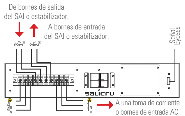
Fig. 8. Ejemplo conexasionado bypass manual de 6 y 10 kVA.
