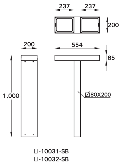
LIGHT LINEAR PT 2 BOLLARD
