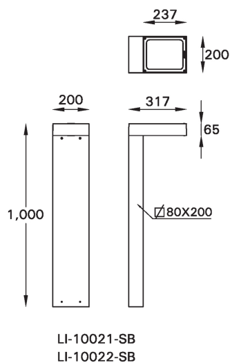
LIGHT LINEAR PT 1 BOLLARD
