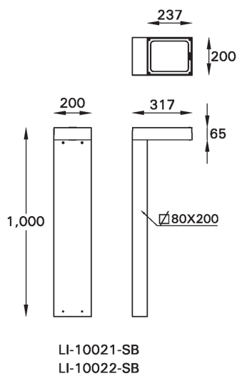
LIGHT LINEAR PT 1 BOLLARD
