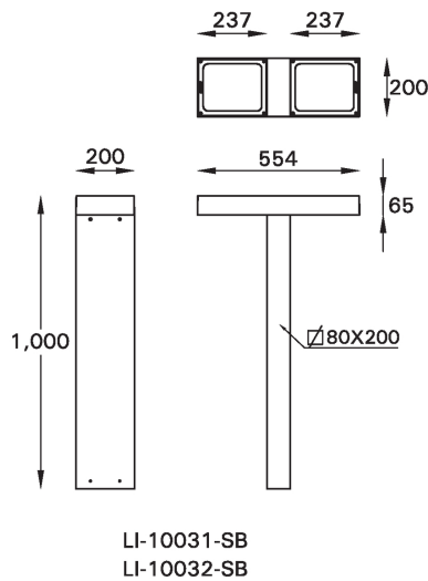
LIGHT LINEAR PT 2 BOLLARD
