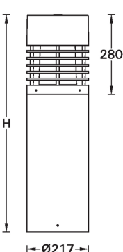
DU-10216-2 DU-10226-2
