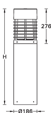
DU-10196-2 DU-10206-2
