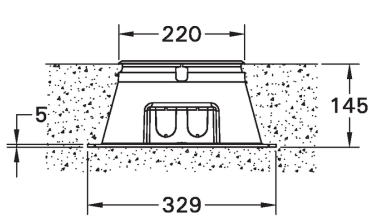
EMBOSS FRAME KI-60485
