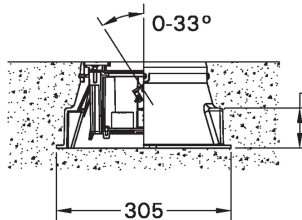
EMBOSS FRAME KI-60485
