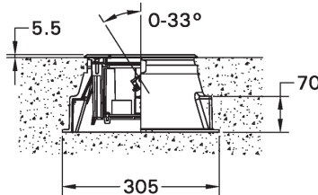
EMBOSS FRAME KI-60485
