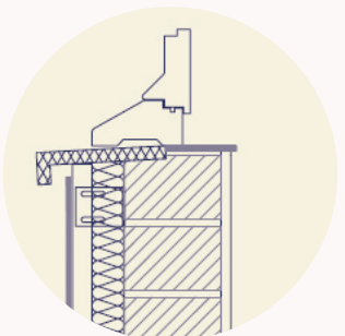
Carpintería Exterior Eliminación Puente térmico
