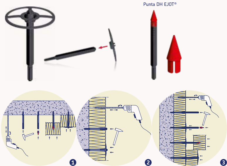
Anclaje DH dos pieza EJOT®
