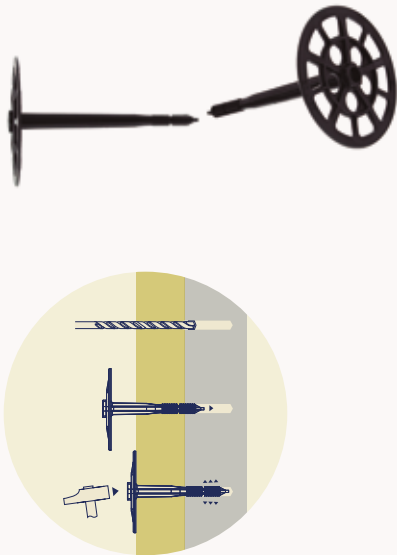
Anclaje CB SPIT
