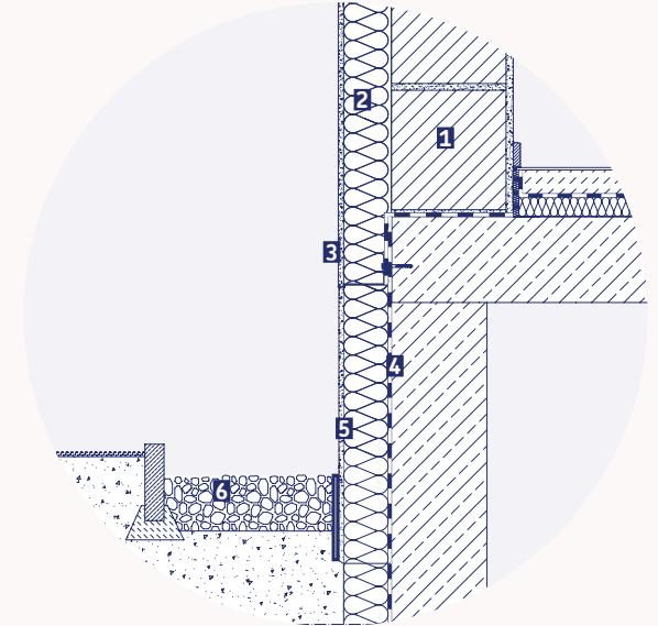
Solución aislamiento exterior
