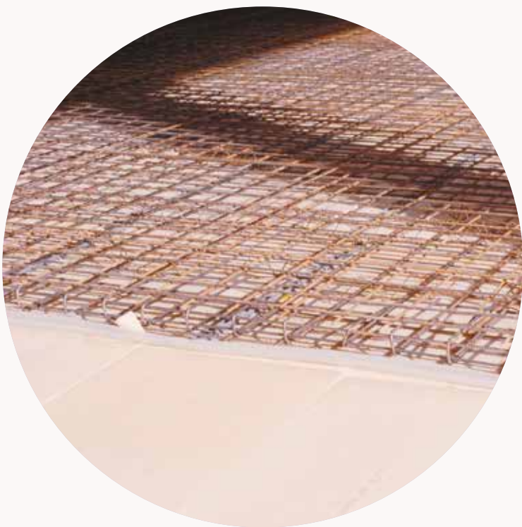
Solución aislamiento bajo suelo radiante
