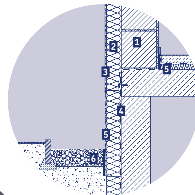
1. Pared exterior 2. URSA XPS F N-III L 3. Revestimientos de fachada 4. Pared exterior del sótano 5. Sellado 6. Base de grava
