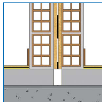
Encontro de divisória assente sobre betonilha
