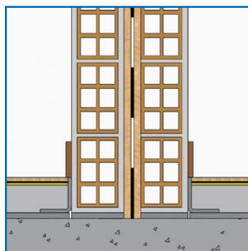
Encontro de divisória assente sobre banda Dessolidarizador de muros
